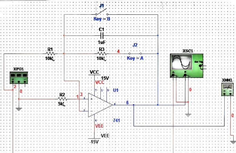
反向积分运算电路
