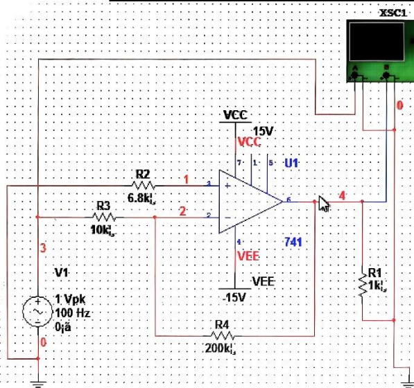
反向比例运算电路
