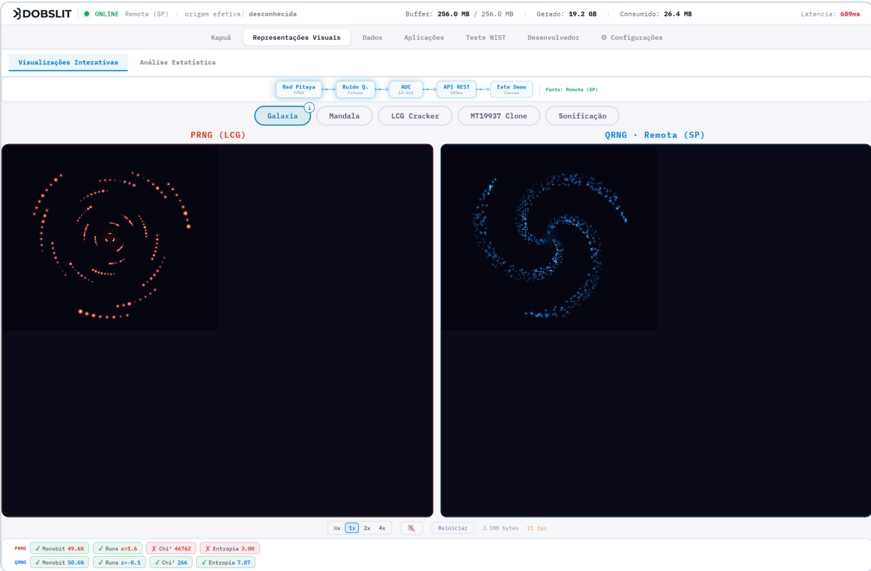
Figura 15 — "Visualizações Interativas → Galáxia": PRNG (LCG, esquerda) com estrutura visível em grade vs QRNG (direita) com espiral suave. Rótulo "QRNG · Remota (SP)" e badges (PRNG reprova Chi²/Entropia; QRNG passa).
