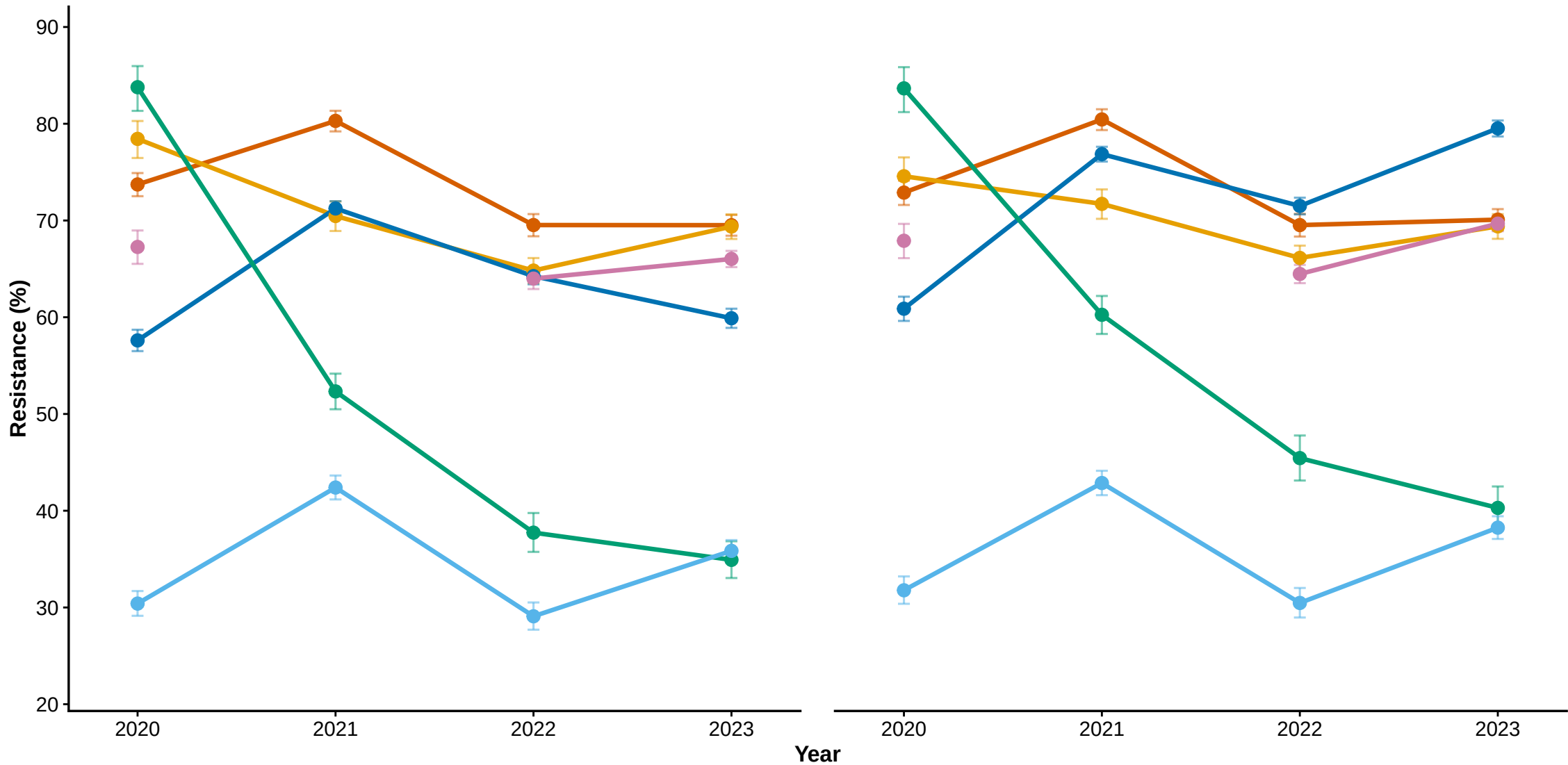
Meropenem
