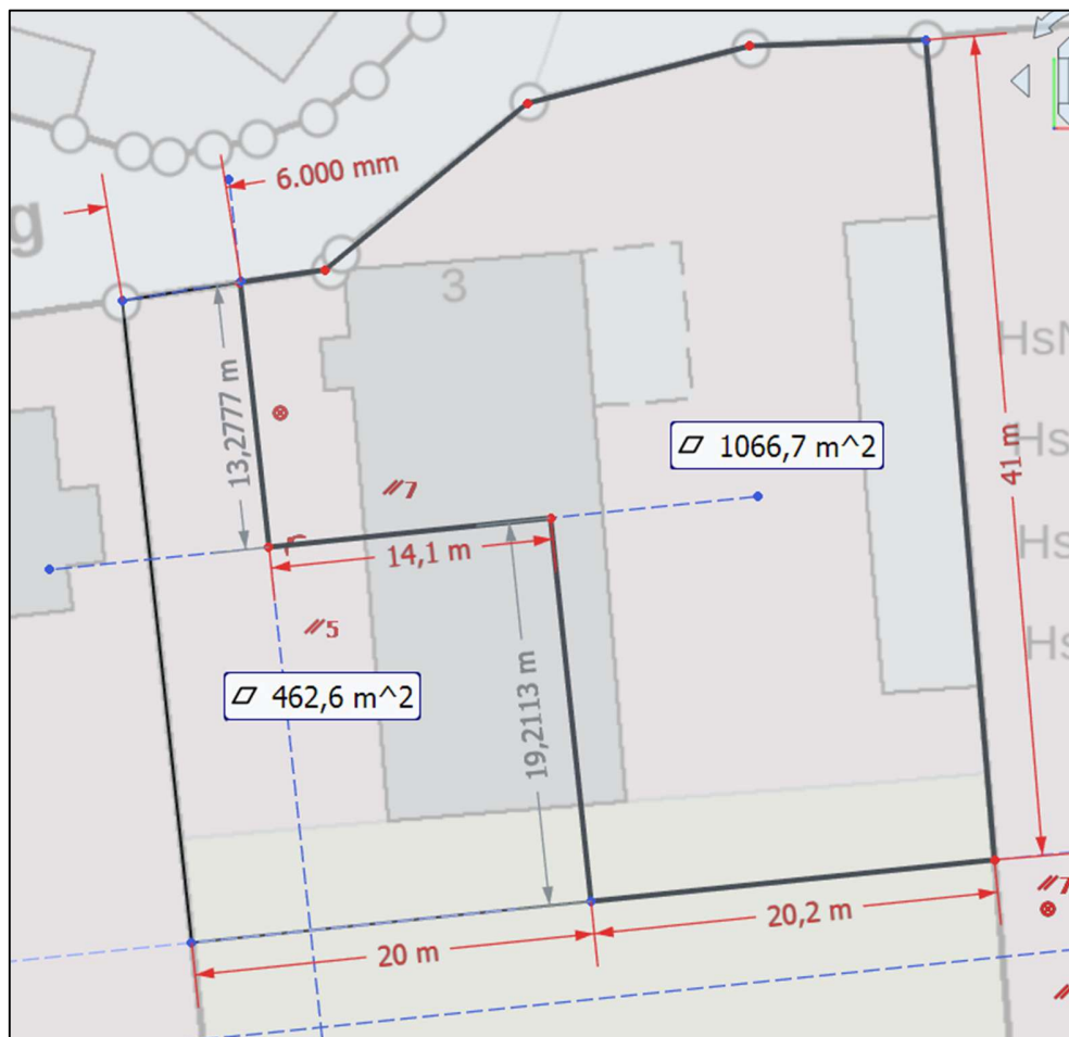
Grundstücksteilung_6_13_20 – Darstellung des Grundstücks im aktuellen Planstand
