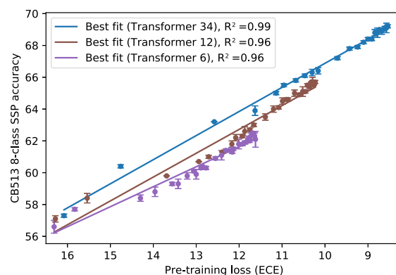
图 S4. 八类二级结构预测准确度与预训练 ECE 的关系。使用 Transformer 模型的特征，在 UR50/S 上进行预训练的过程中训练一个深度二级结构预测器。使用 Netsurf 训练序列和 CB513 测试集。绘制了每个预训练检查点的下游模型三个种子的平均值，并为每个 Transformer 绘制了最佳拟合线。
