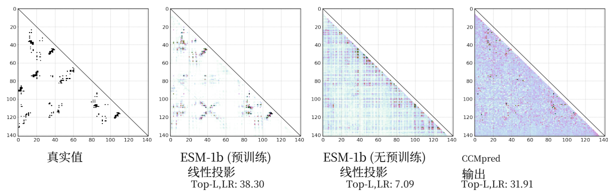
(d) d3ddja1 (CBS域对) (141 残基)
