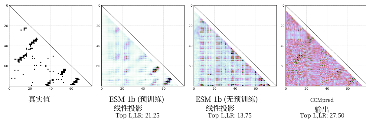
(a) dlbc01 (mu 转座酶, C-末端结构域) (80 残基)
