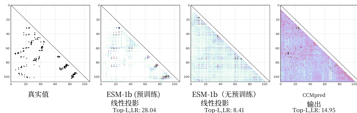
(c) dl192a1 (皮质亚单位) (107 残基)
