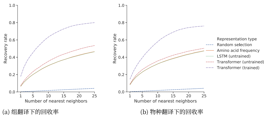
图 S1. 学习到的序列表示可以在同源组和物种之间进行翻译。图中显示了在 (a) 同源组翻译和 (b) 物种翻译下最近邻搜索的回收率。在这两种设置中, 训练的变换器表示空间具有更高的回收率。结果显示为在 UniParc 上预训练的 36 层变换器。为了定义同一物种的蛋白质 a 和蛋白质 b 之间的线性翻译, 我们将源集和目标集定义为 24 种不同物种中蛋白质 a 或蛋白质 b 的平均值。如果表示空间线性编码同源性, 那么将这些平均值的差添加到某种物种的蛋白质 a 将能够恢复同一物种中的蛋白质 b 。我们使用类似的方法将源物种 s 的蛋白质翻译为目标物种 t 中的同源物。在这里, 我们考虑 s 和 t 中蛋白质的平均表示。如果表示空间按物种线性组织, 那么将平均表示的差添加到物种 s 中的蛋白质将恢复物种 t 中对应的蛋白质。
