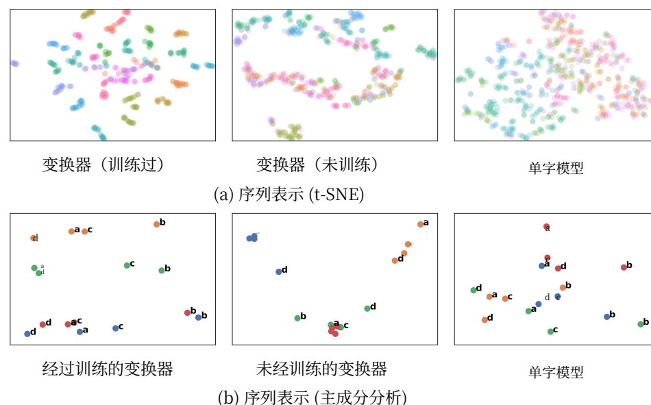
图 2. 蛋白质序列表示编码并组织生物变异。(a) 每个点代表一个基因, 且每个基因的颜色由其所属的同源组决定(维度通过 t-SNE 降维)。经过训练的表示空间中, 同源基因组聚集得很密集。相反, 未经训练的表示空间和单字模型表示并未显示出由进化关系组成的强组织。(b) 在经过训练的表示空间中, 对应于共同生物变异的基因线性相关。基因的颜色由其同源组决定, 物种由字符标签表示。主成分分析在经过训练的表示空间中恢复了物种轴(水平)和同源轴(垂直), 但在未经训练或单字模型空间中未能恢复。表示来自于在 UniParc 上训练的 36 层 Transformer 模型。
