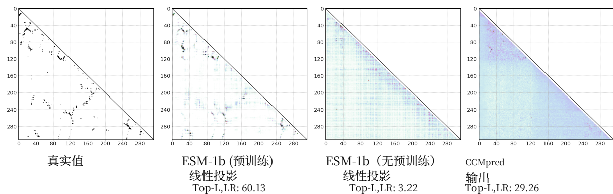
(f) d4jnca1 ( \alpha/\beta -水解酶) (311 残基)
