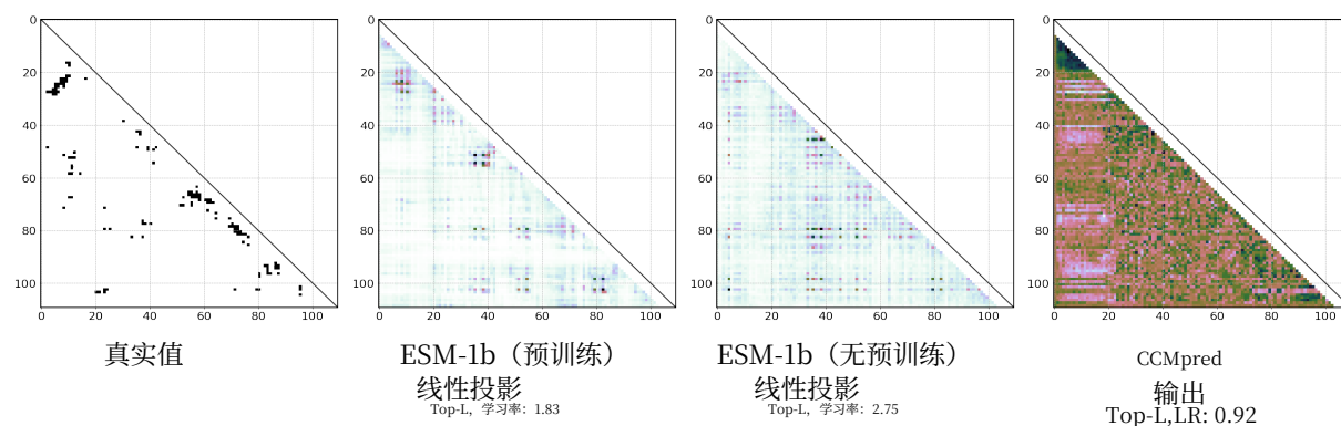
(b) dlgyoa (多血红素细胞色素) (109 残基)
