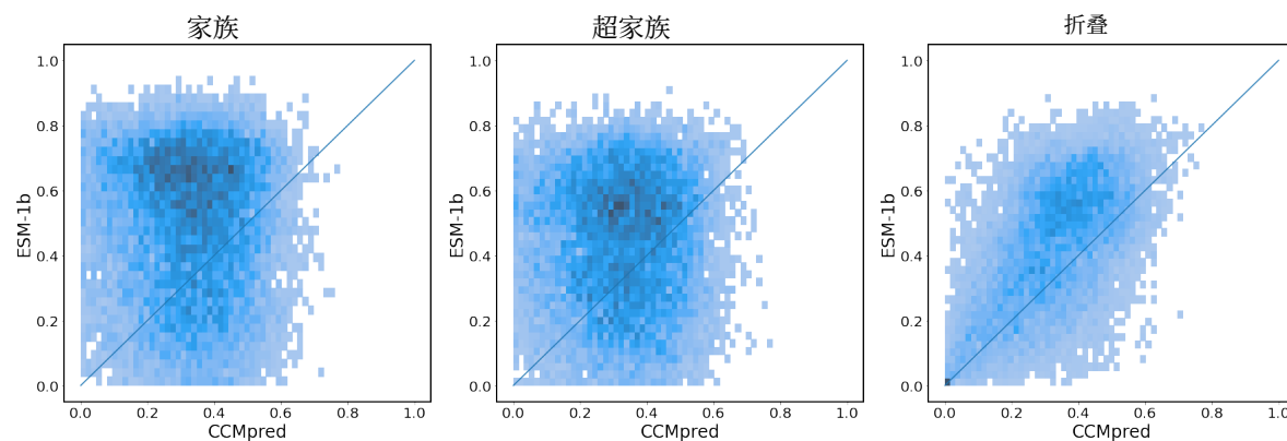
(b) 线性投影 ESM1-b 与 CCMpred
