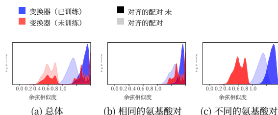
图 3. 经过训练的模型产生的最终表示隐式对序列进行对齐。余弦相似度分布显示了来自PFAM家族PF01010中的序列的残基的最终表示。对齐 (深蓝色) 和未对齐 (浅蓝色) 分布之间的差异暗示训练后的
