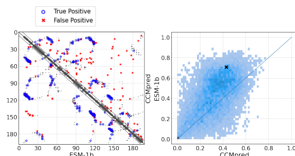
图 5. 残基-残基接触（线性投影）。左侧：对保持折叠水平示例d1n3ya_的Top-L预测，具有vWA样折叠。真正阳性以蓝色显示，假阳性以红色显示，叠加在灰色的真实接触图上。ESM-1b 变换器的投影位于对角线下方，CCMpred的预测位于对角线上方。右侧：精确度分布（Top-L远程），在五个测试分区内比较ESM-1b投影与CCMpred，结构保持在折叠水平。可视化域标记为x。
