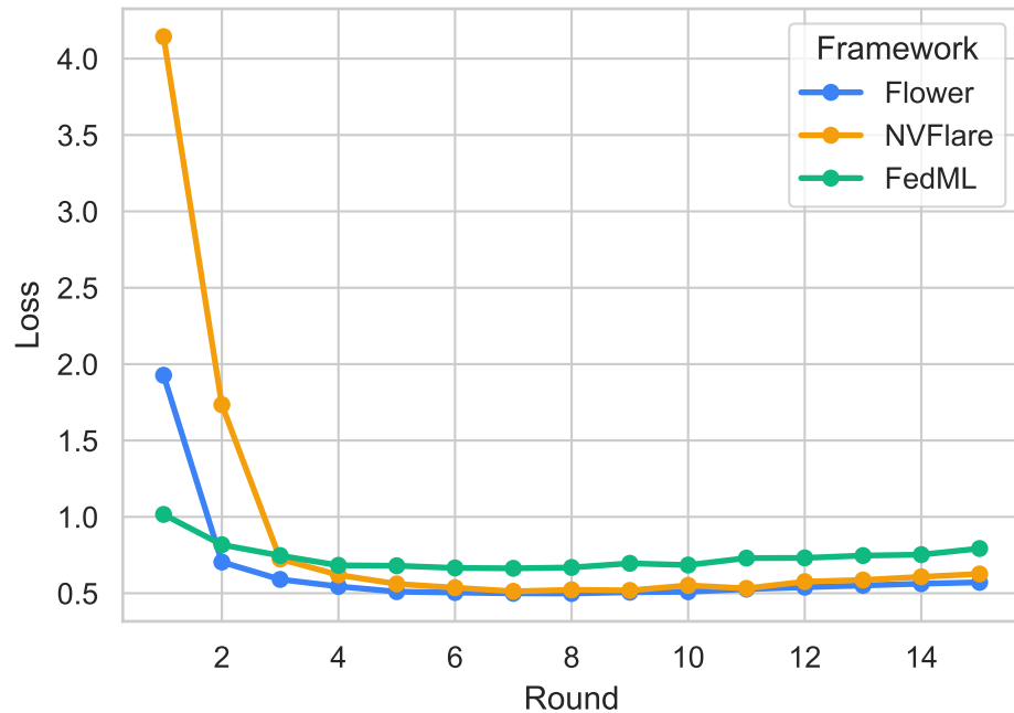
Loss per round
