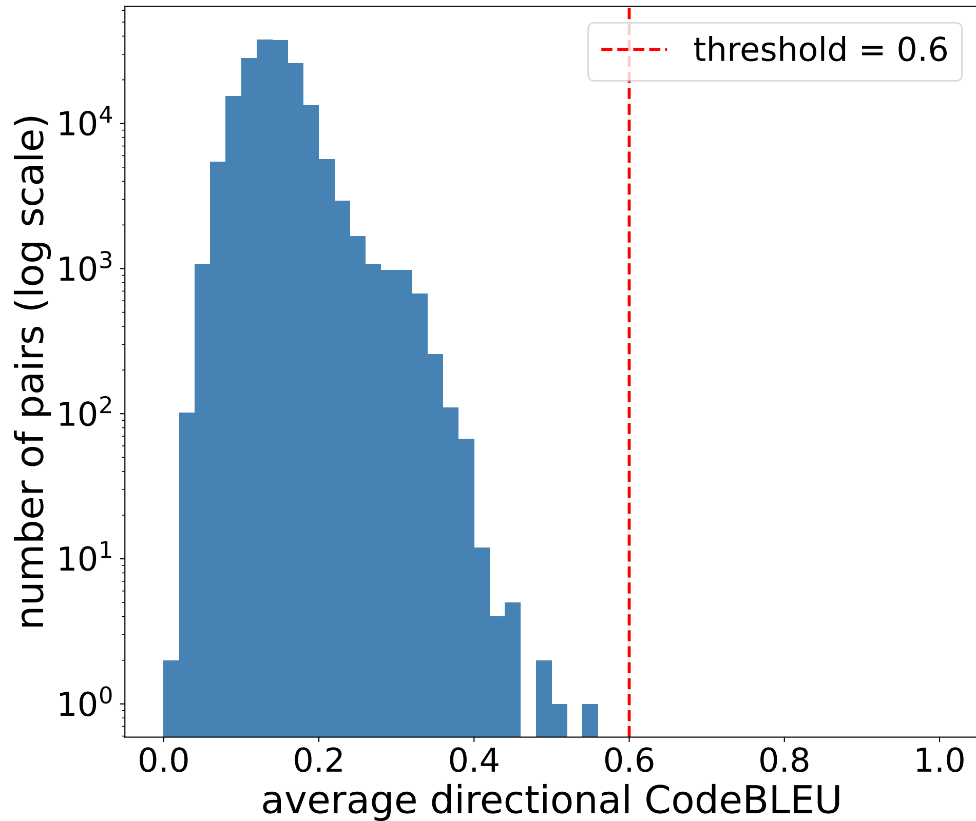
Pairwise CodeBLEU distribution
