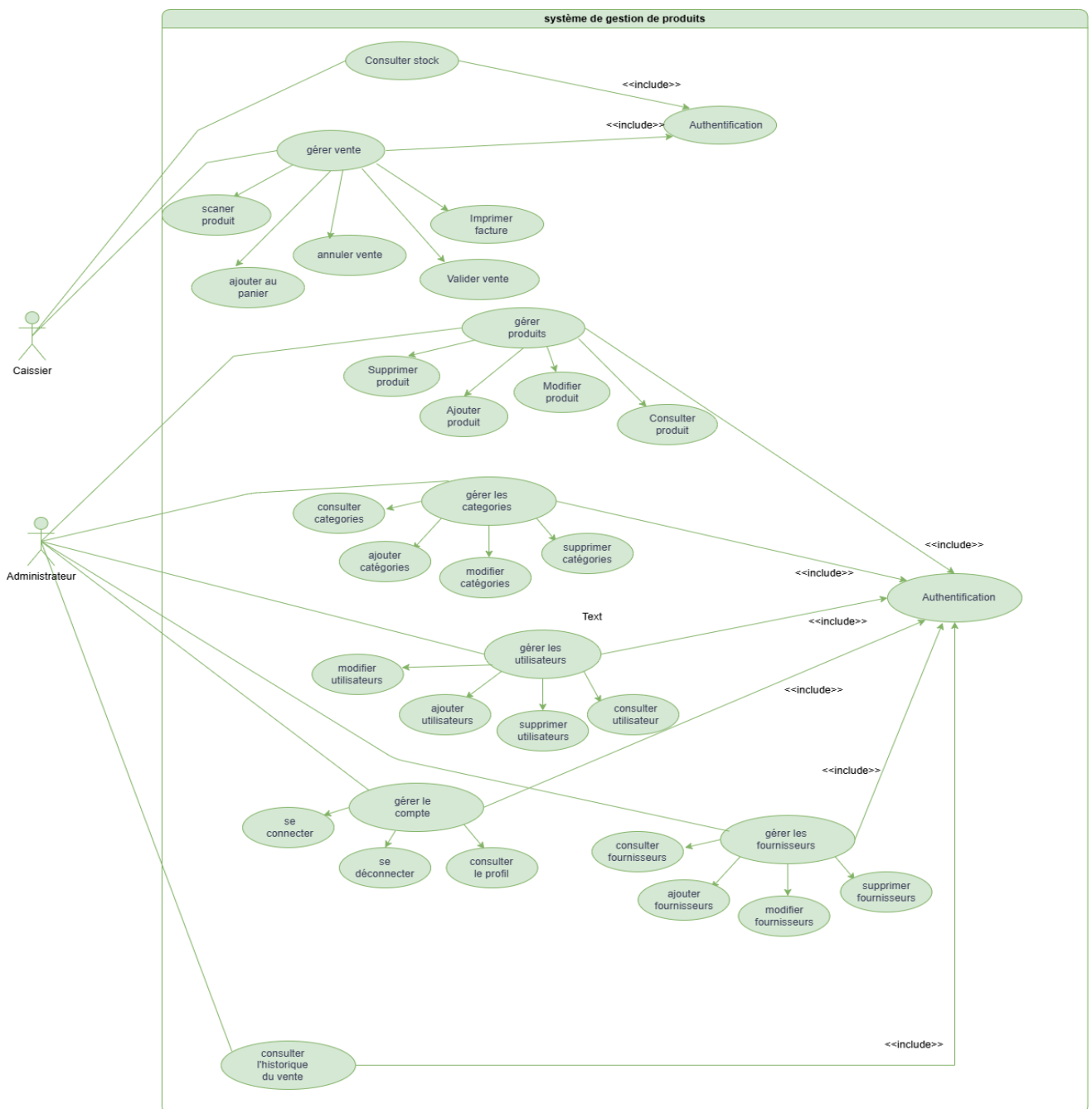
Figure 3. 4 Diagramme de cas d'utilisation
