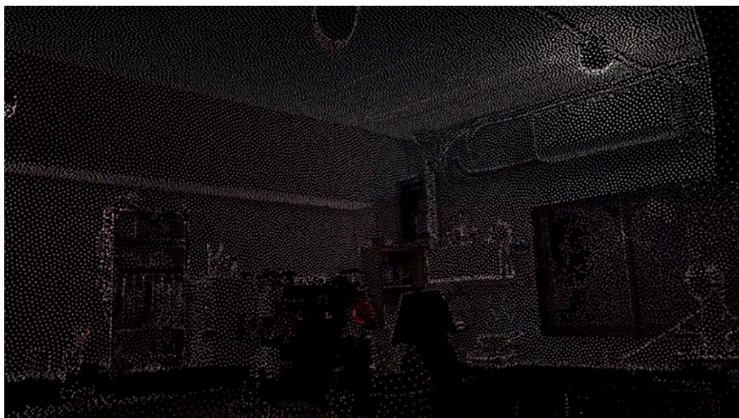
단안(單眼) LiDAR 로 한 자리에서 스캔된 카페 내부의 포인트 클라우드. 의도적으로 협소한 시야를 드러낸다.
