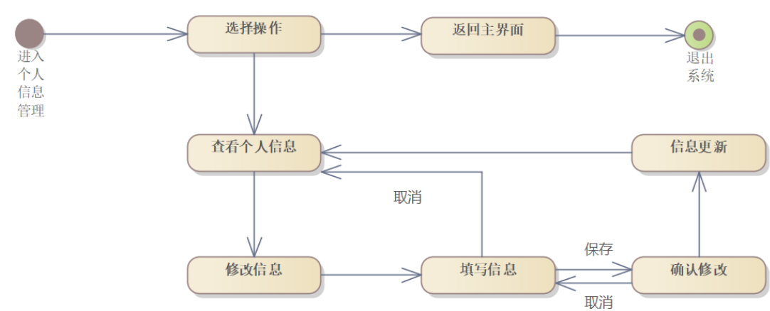
图 42 用户个人信息处理状态图
