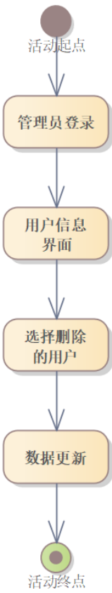
图 9 删除用户活动图
