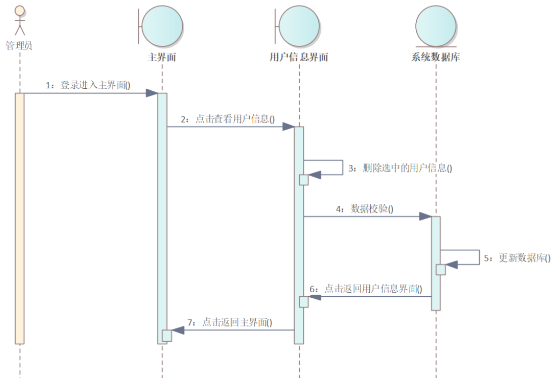
图 23 删除用户信息顺序图
