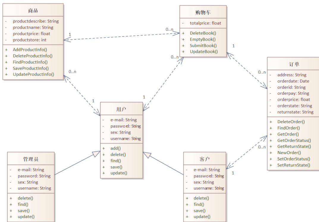
图 17 类的总关系图
