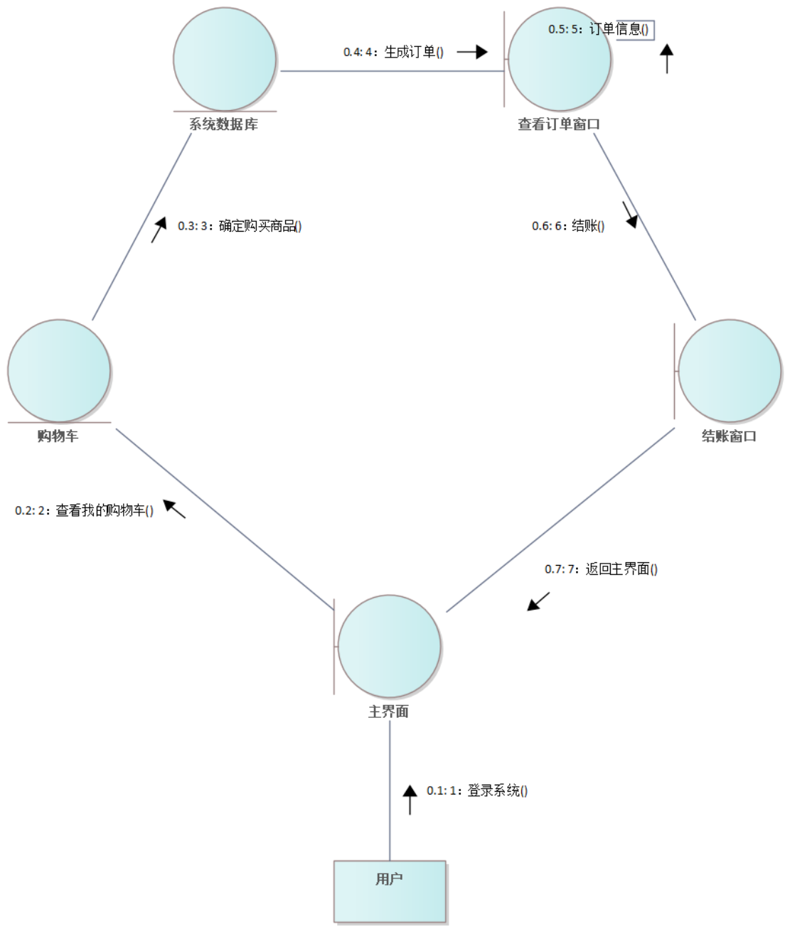
图 39 常规订单处理协作图
