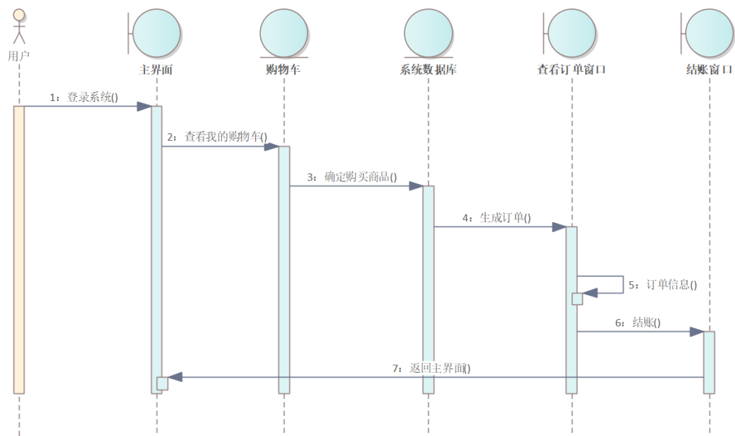
图 28 常规订单处理顺序图
