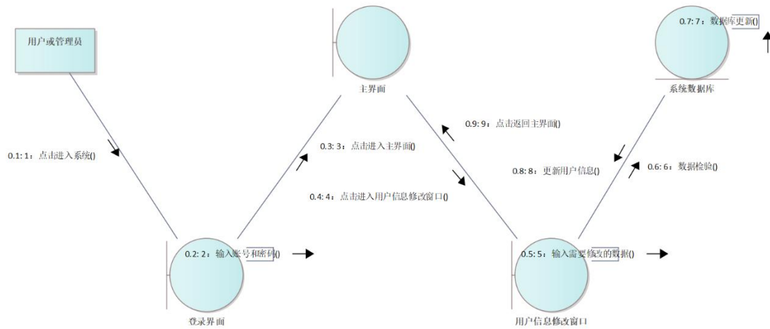
图 32 修改用户信息协作图
