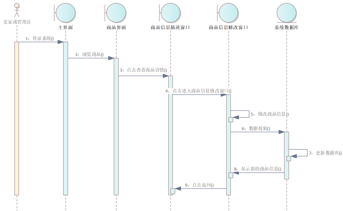
图 25 修改商品信息顺序图
