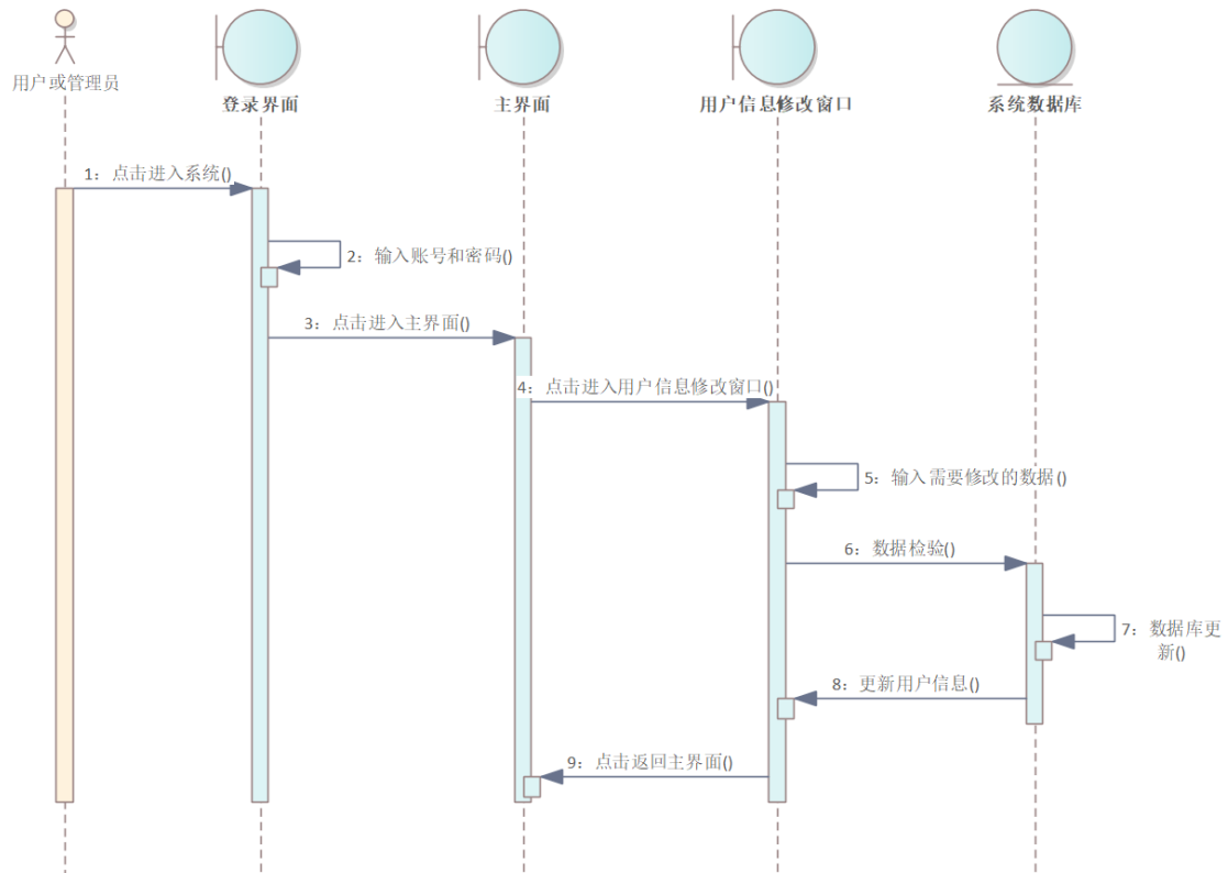
图 21 修改用户信息顺序图
