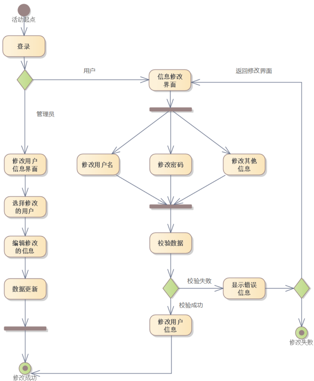
图8 修改用户活动图
