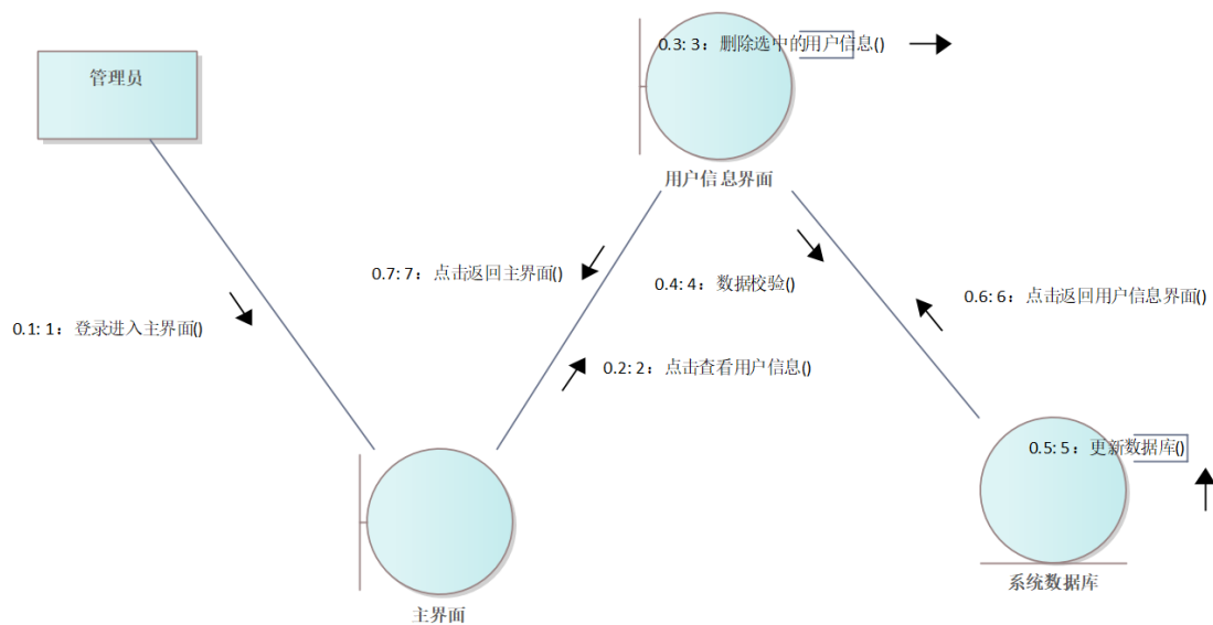
图 34 删除用户信息协作图
