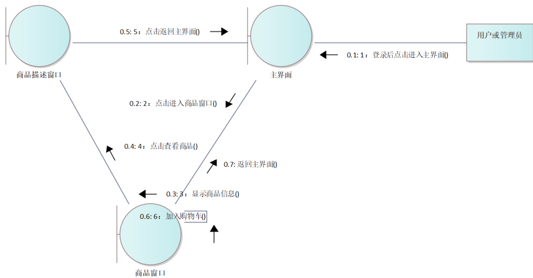
图 35 查看商品信息协作图
