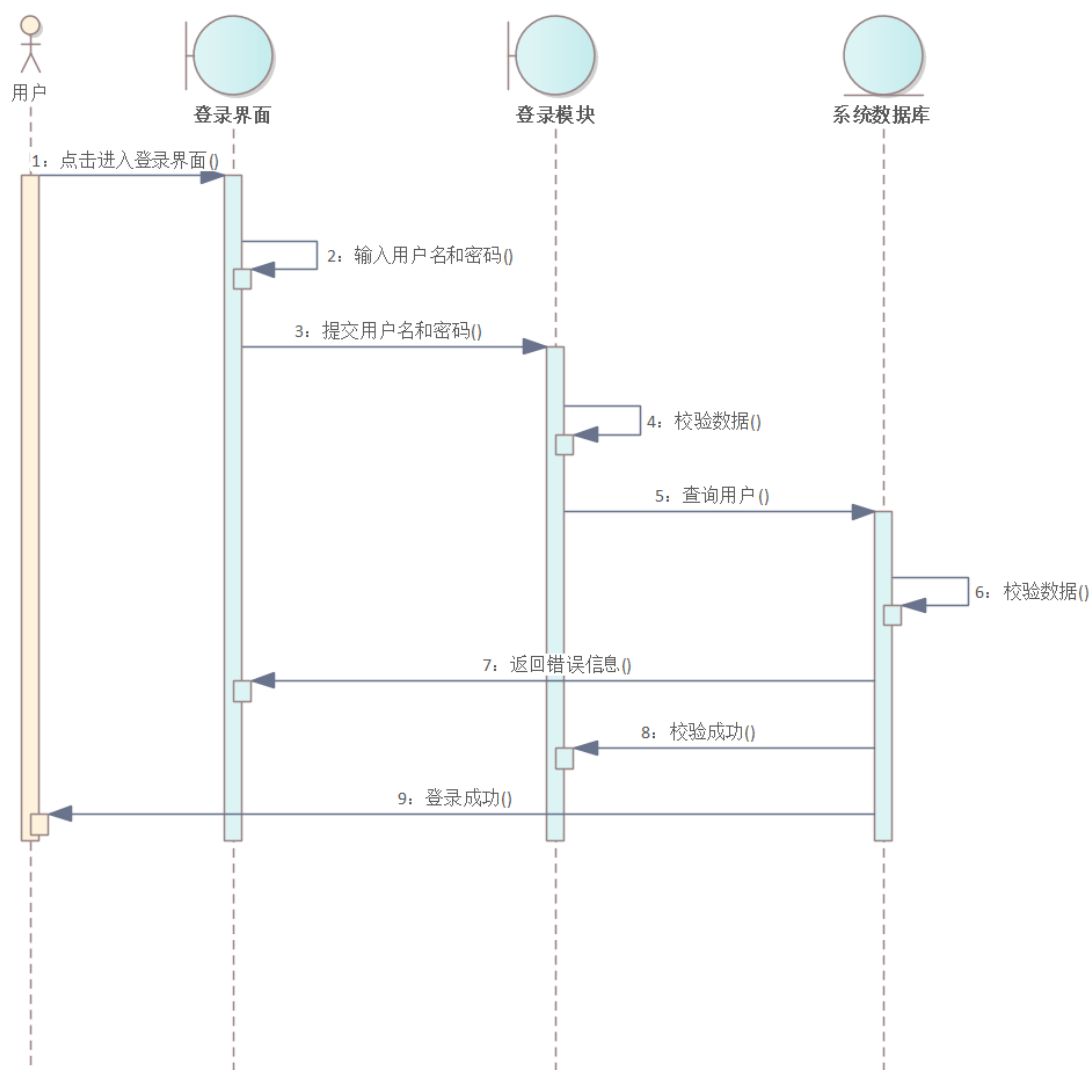
图 20 登录顺序图
