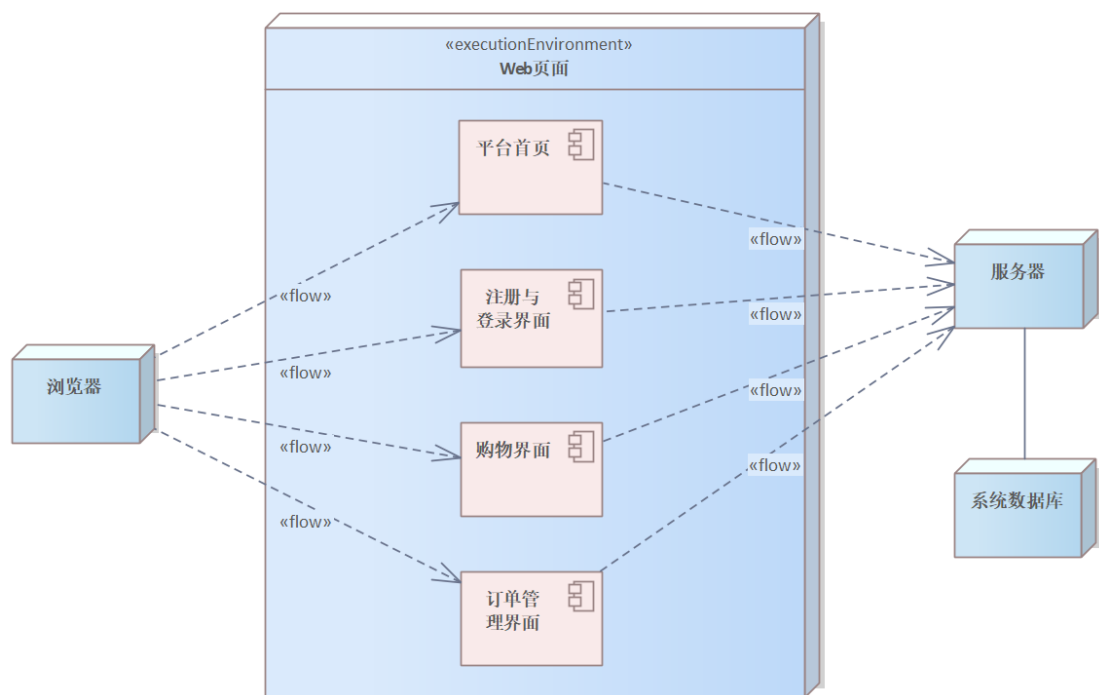
图 49 部署图
