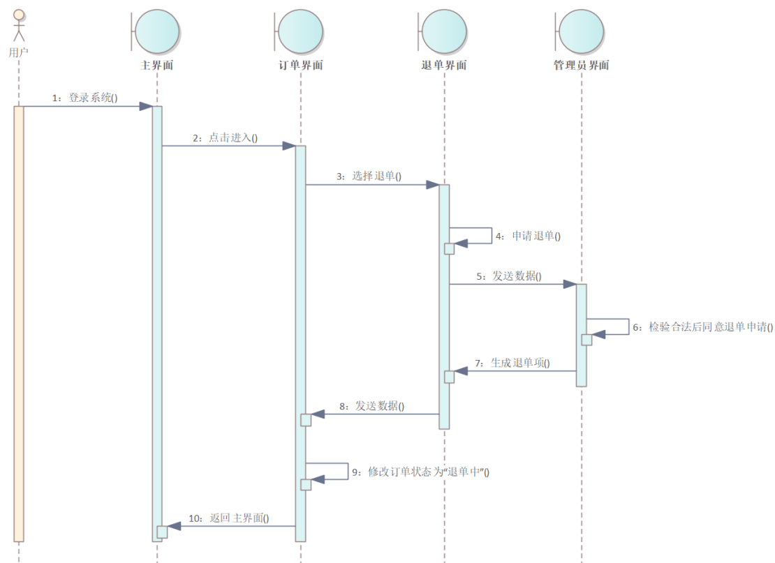
图 29 退货订单处理顺序图
