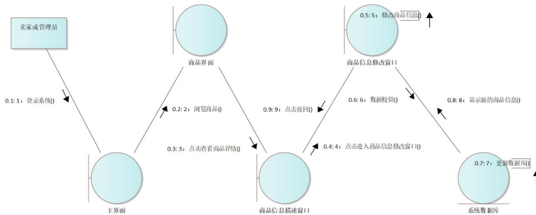
图 36 修改商品信息协作图
