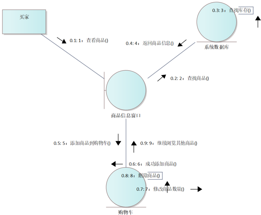
图 38 购买商品协作图
