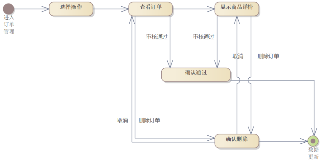
图 46 用户订单处理状态图
