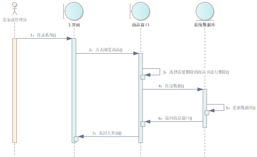
图 26 删除商品信息顺序图
