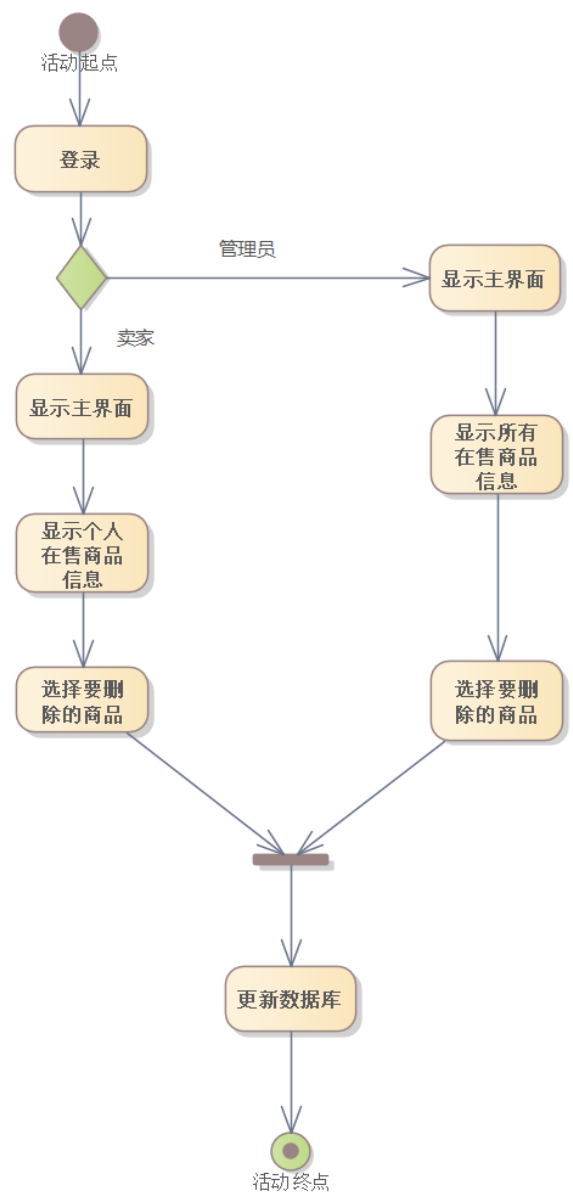
图 13 删除商品信息活动图
