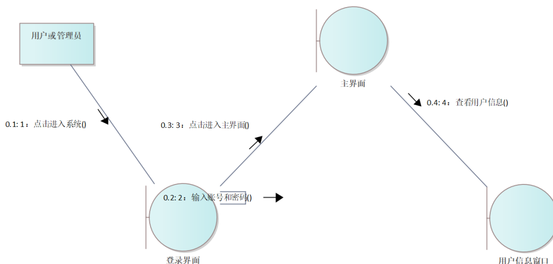
图 33 查看用户信息协作图
