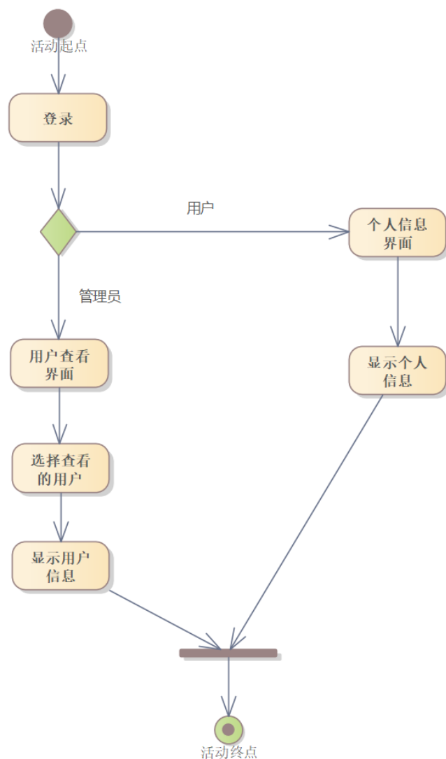
图 10 查看用户活动图
