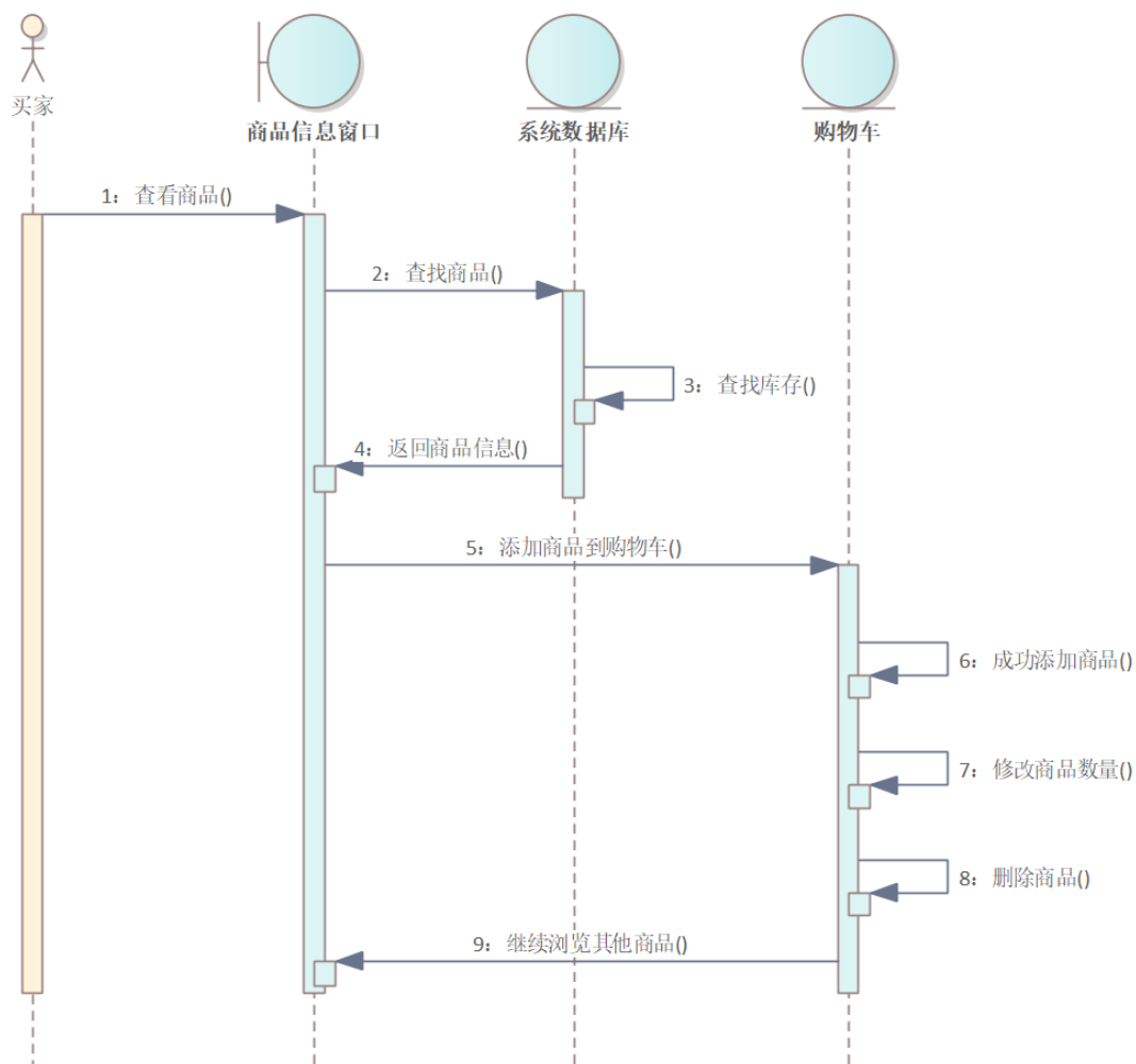
图 27 购买商品顺序图
