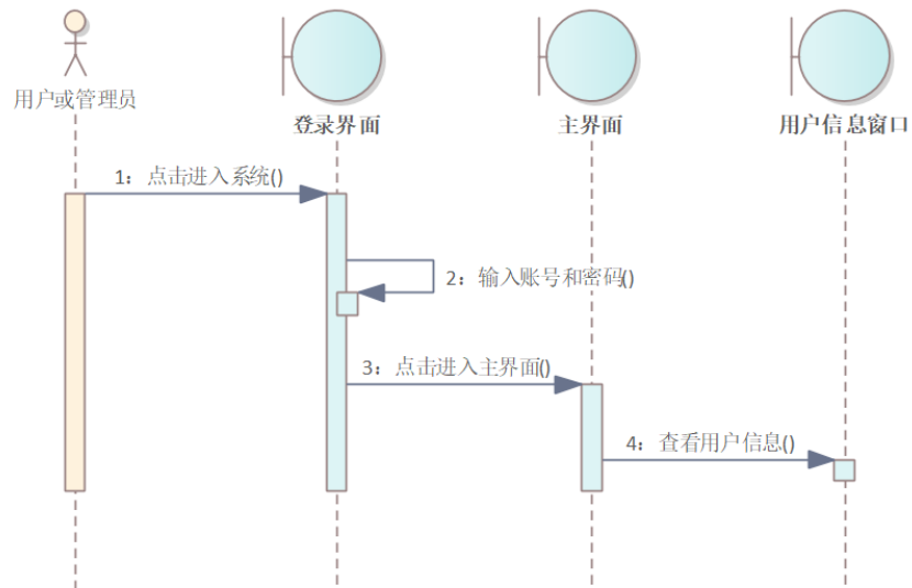
图 22 查看用户信息顺序图
