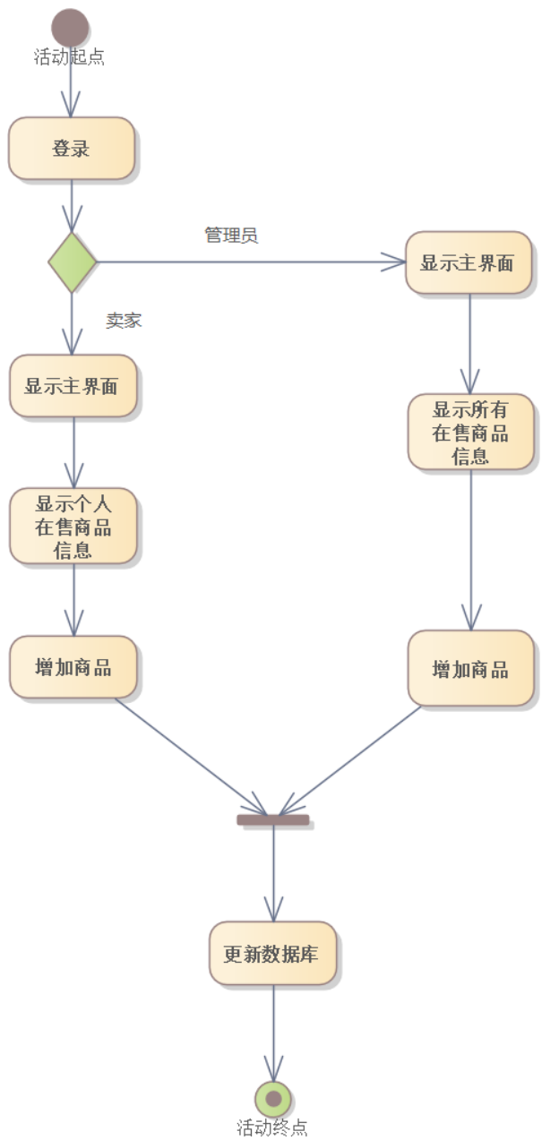
图 14 增加商品信息活动图
