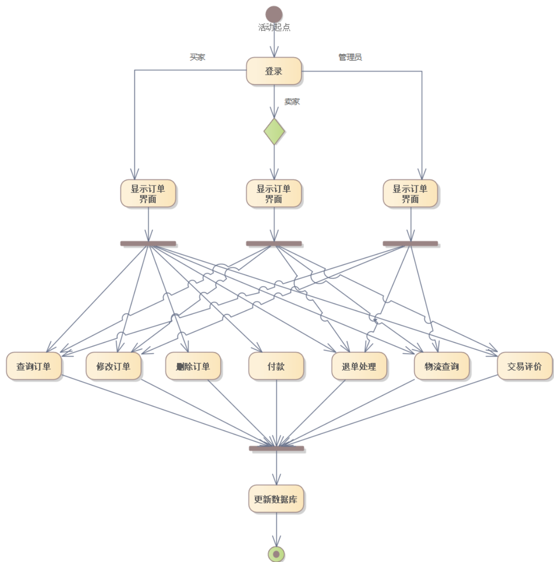
图 16 订单管理活动图
