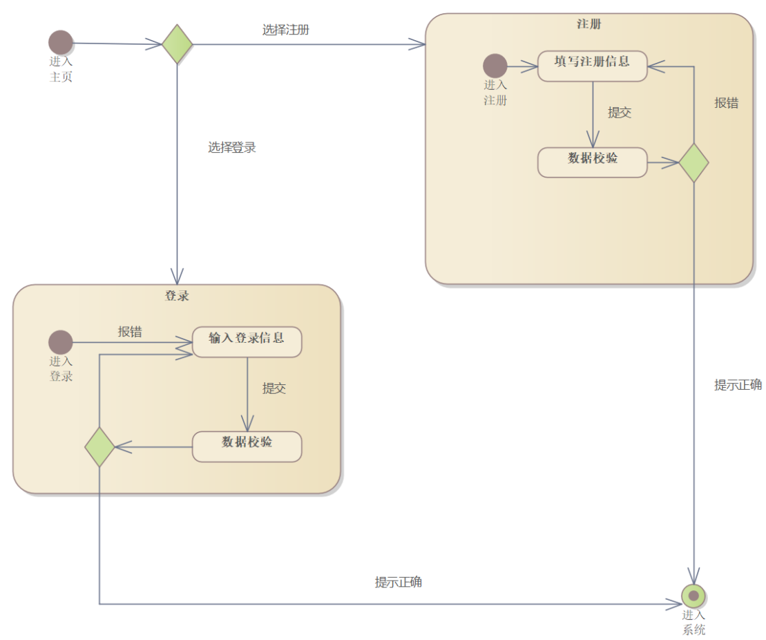
图 41 注册登录状态图
