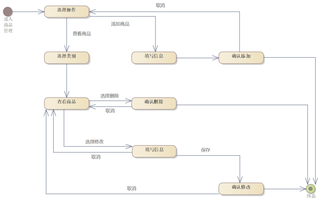
图 47 商品管理状态图
