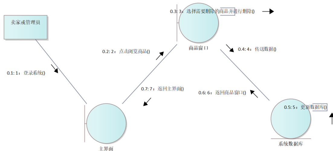
图 37 删除商品信息协作图
