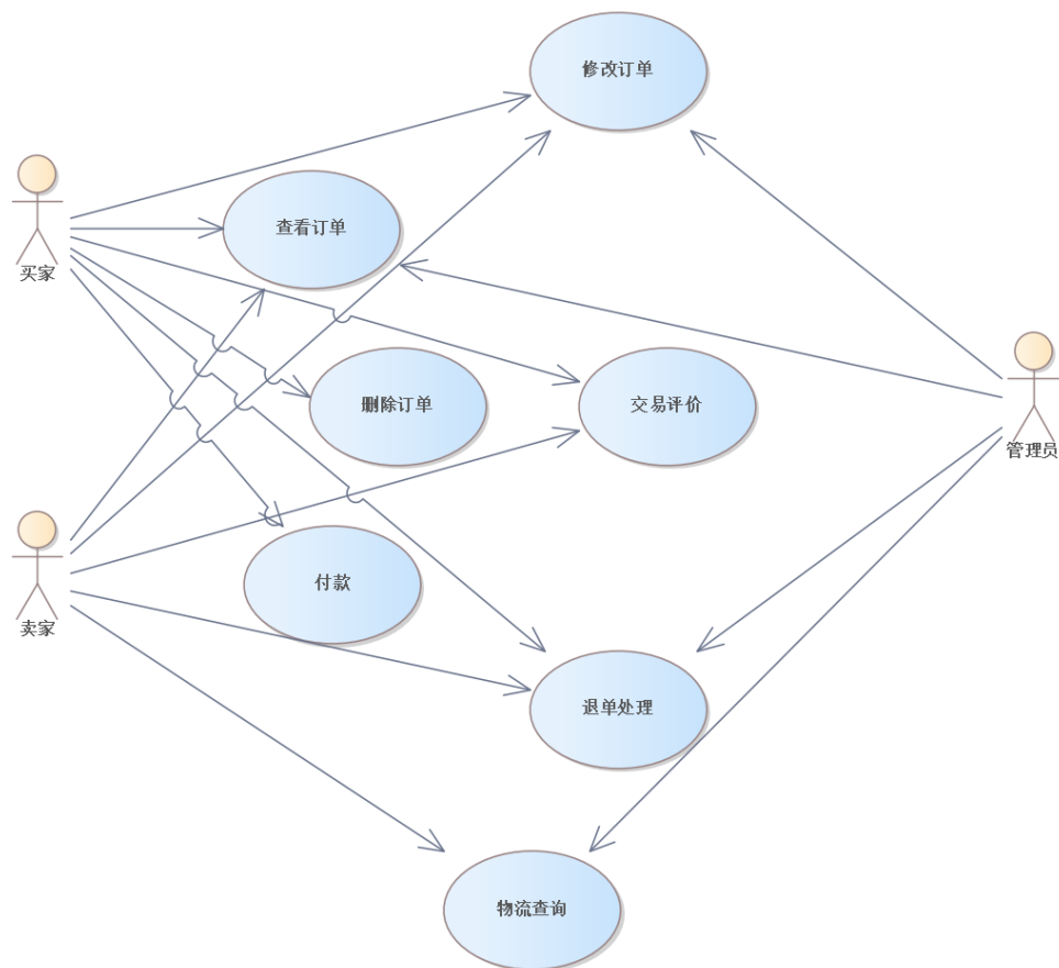
图 5 订单管理用例图
