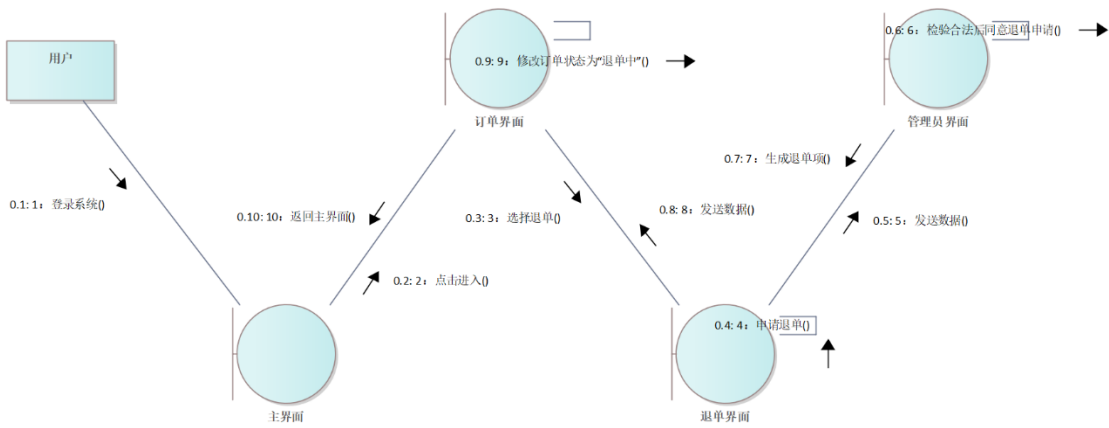
图 40 退货订单处理协作图
