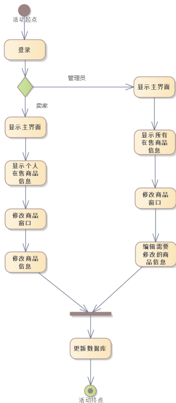
图 12 修改商品信息活动图
