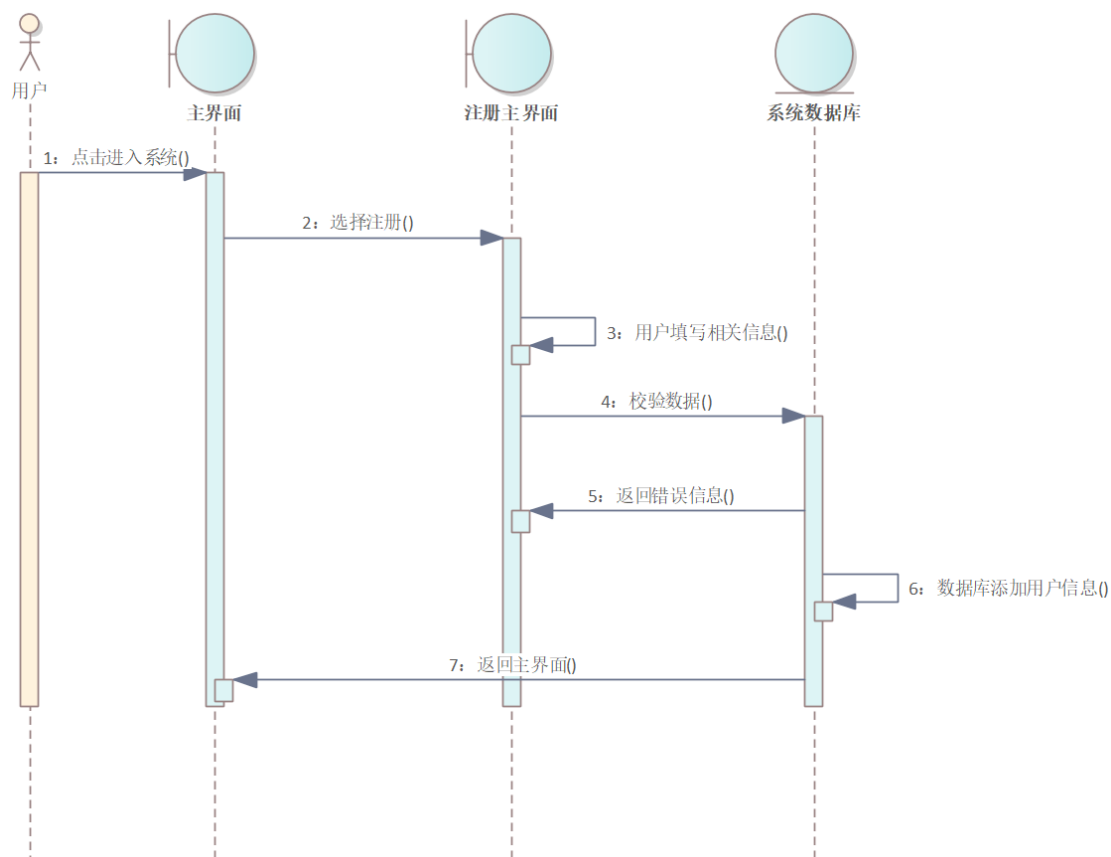
图 19 注册顺序图
