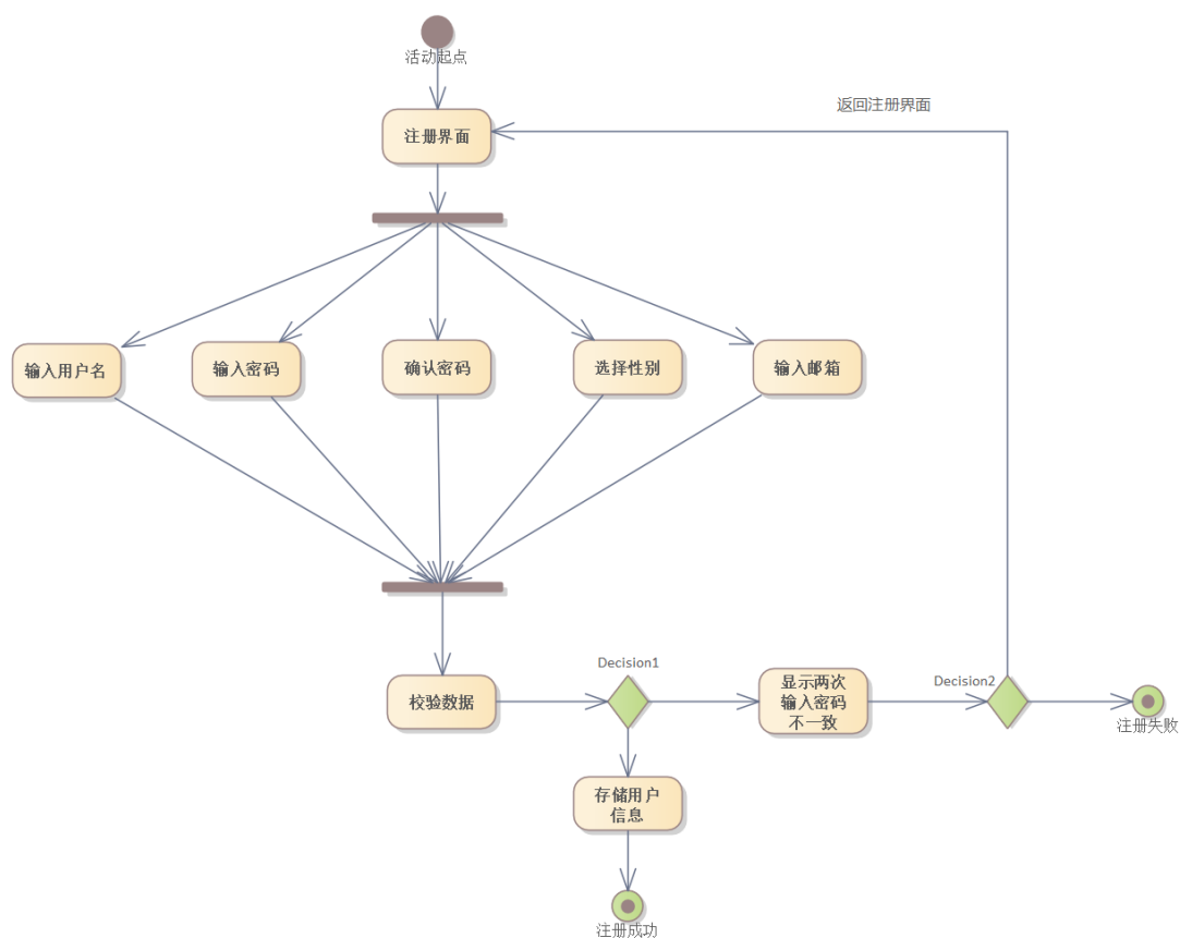
图 6 注册活动图
