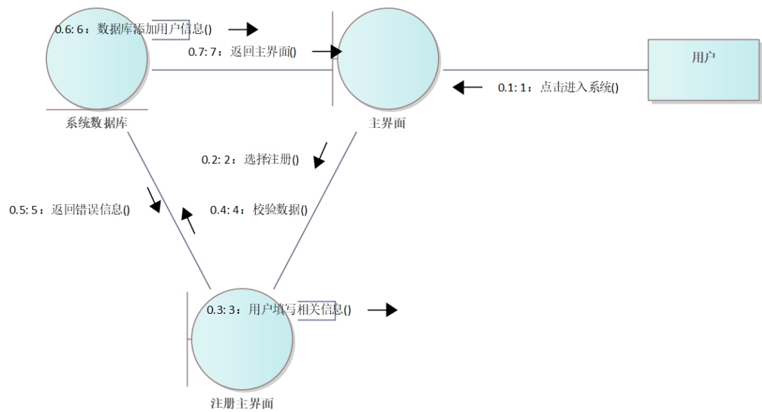
图 30 注册协作图
