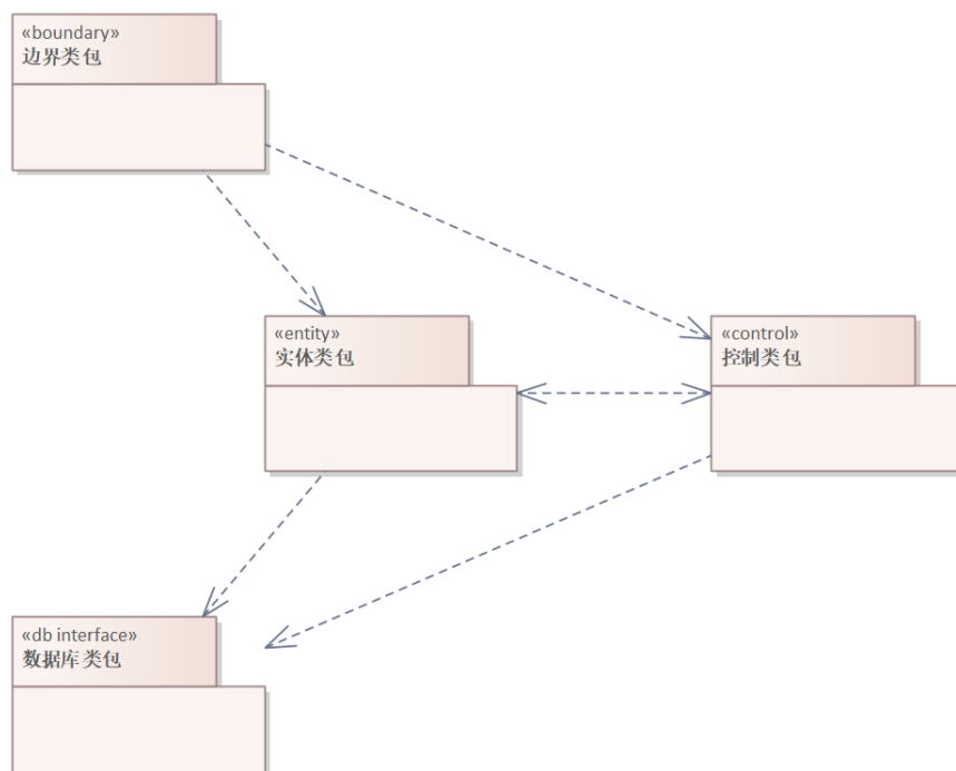
图 18 类的包图
