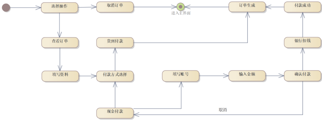
图 44 付款状态图
