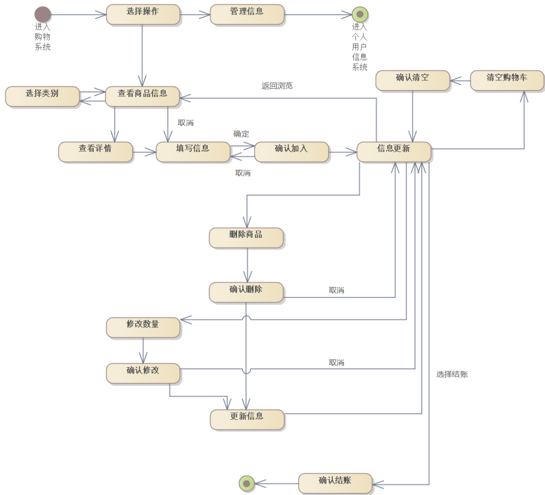
图 43 购物状态图
