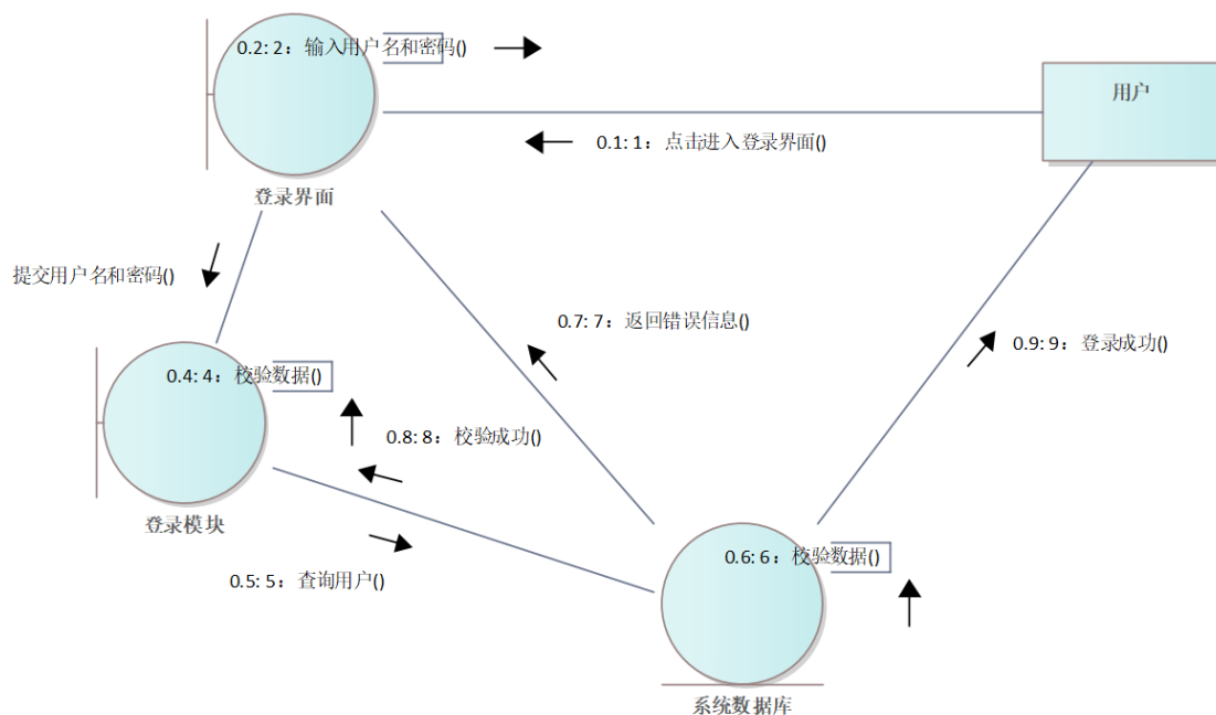
图 31 登录协作图
