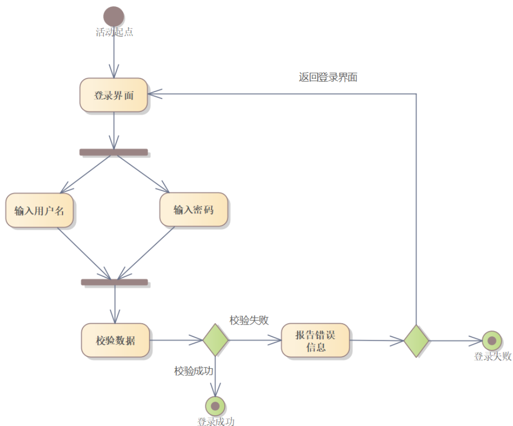
图 7 登录活动图
