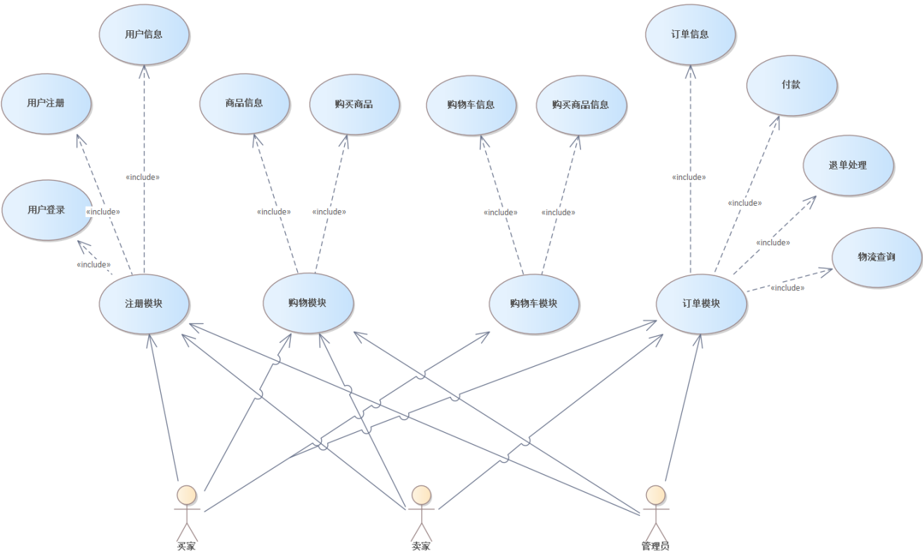
图 1 总用例图
