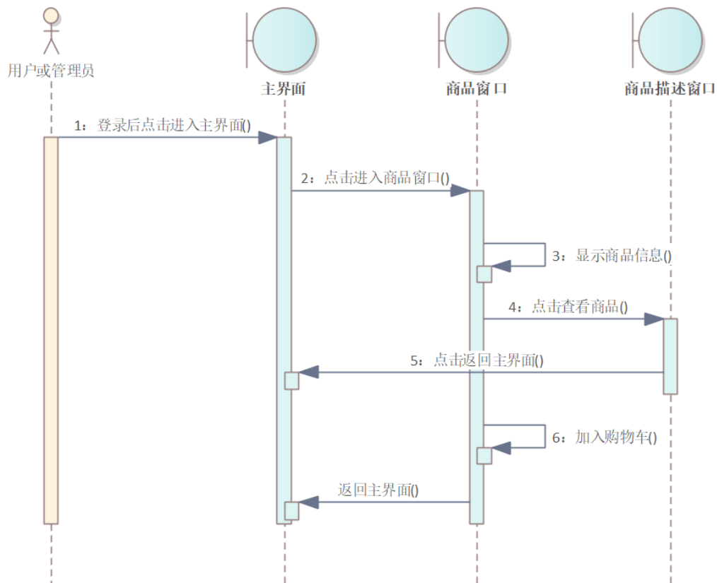
图 24 查看商品信息顺序图
