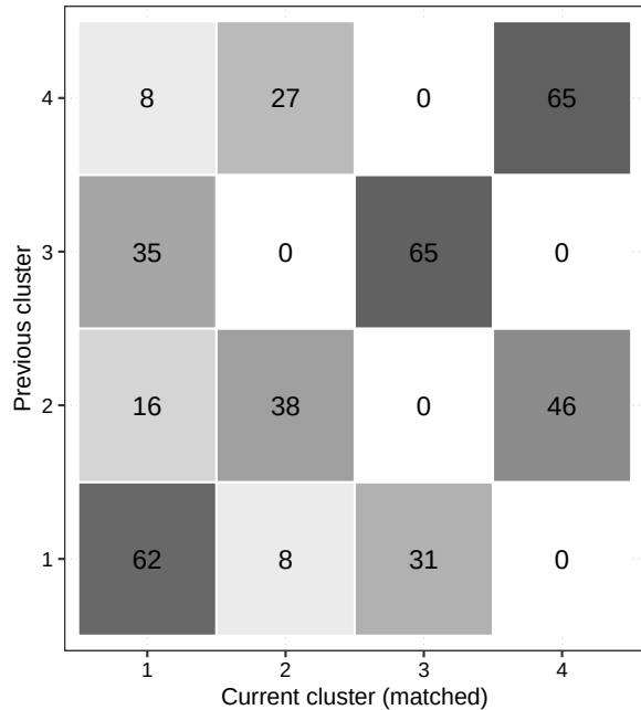
1976 -&gt; 1979 (ARI = 0.233)
