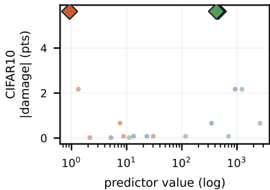
CNN
