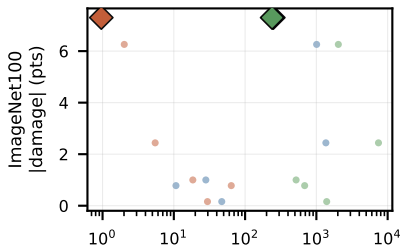
CNN
