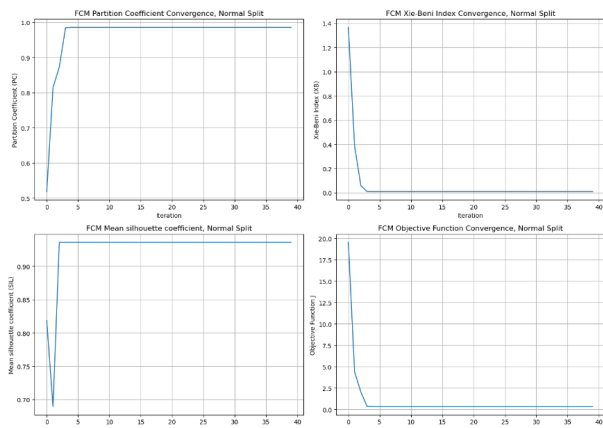
Slika 1: Evalvacijske metrike za FCM
