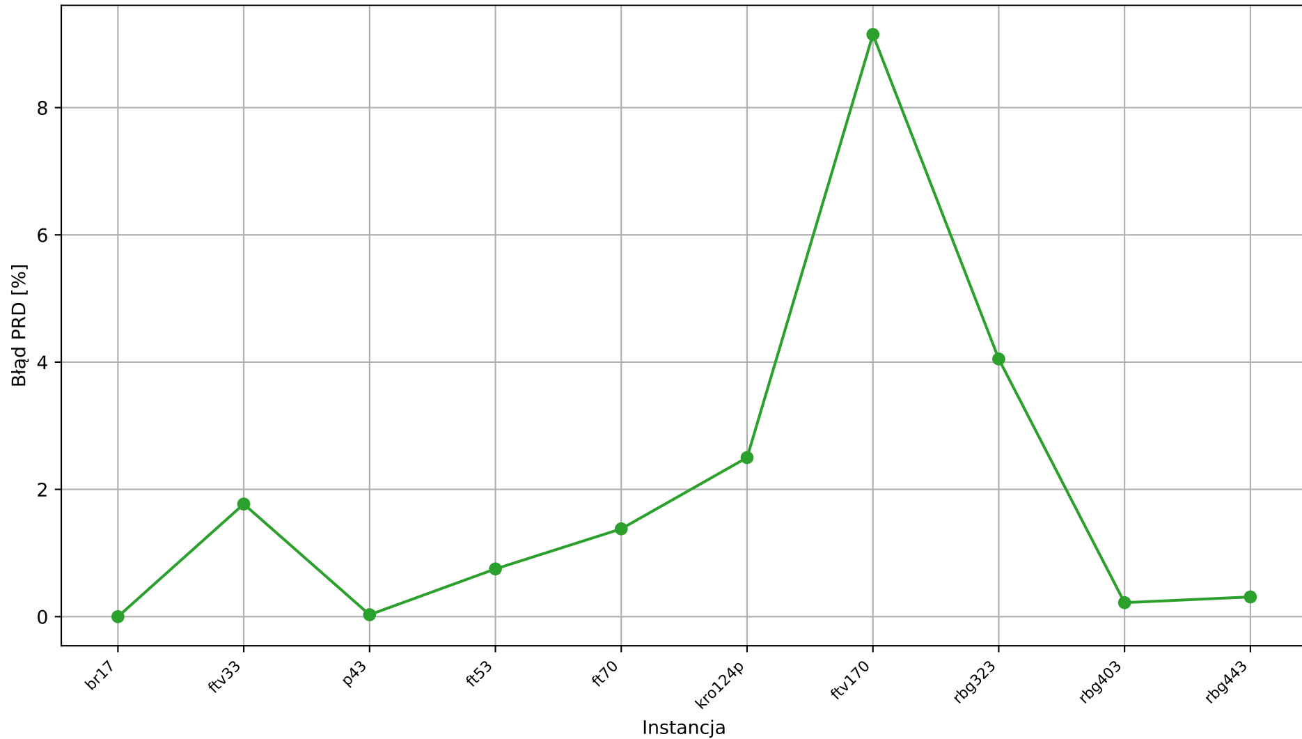
Błąd PRD od rozmiaru instancji
