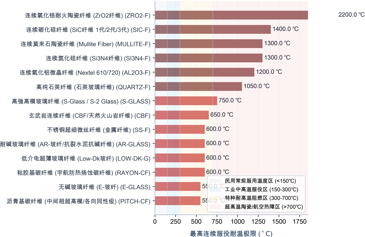
图 1-4 现代化学纤维耐温极限服役温度天花板梯队排行 (Top 14)
