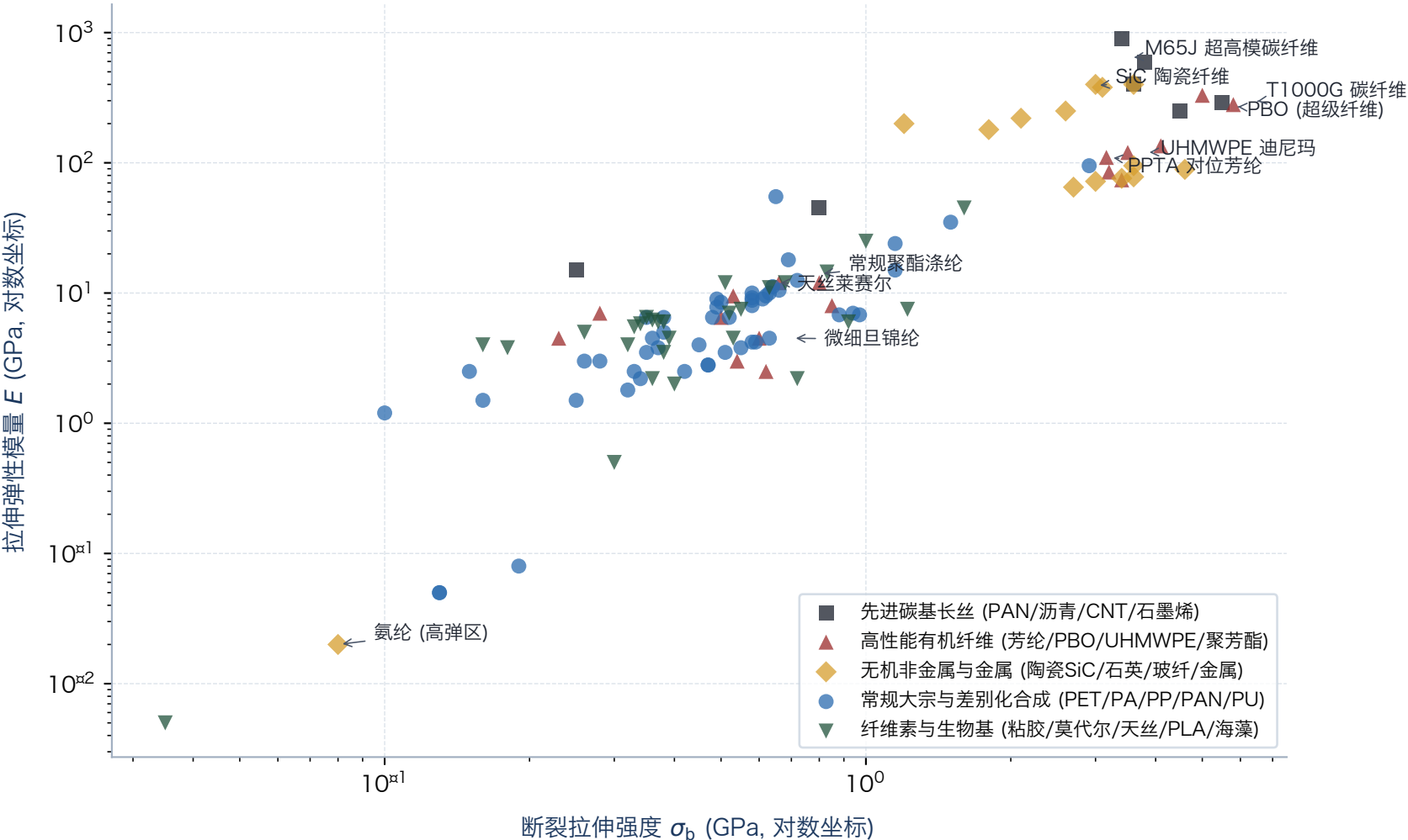
图 1-2 化学纤维拉伸强度与初始模量 Ashby 材料性能图谱
