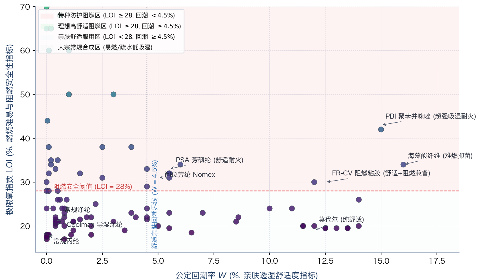
图 1-3 化学纤维公定回潮率 (舒适度) 与极限氧指数 LOI (阻燃安全性) 四象限定位
