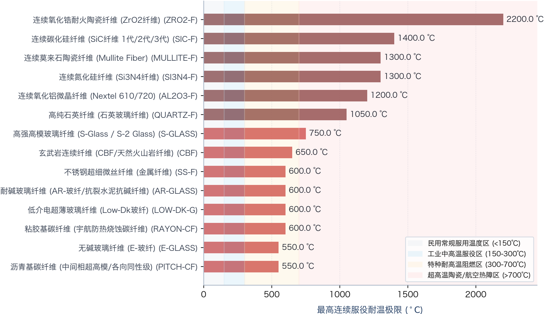
图 1-4 现代化学纤维耐温极限服役温度天花板梯队排行 (Top 14)
