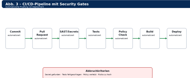
Abb. 3: CI/CD-Pipeline mit Sicherheitsprüfungen und Abbruchkriterien
