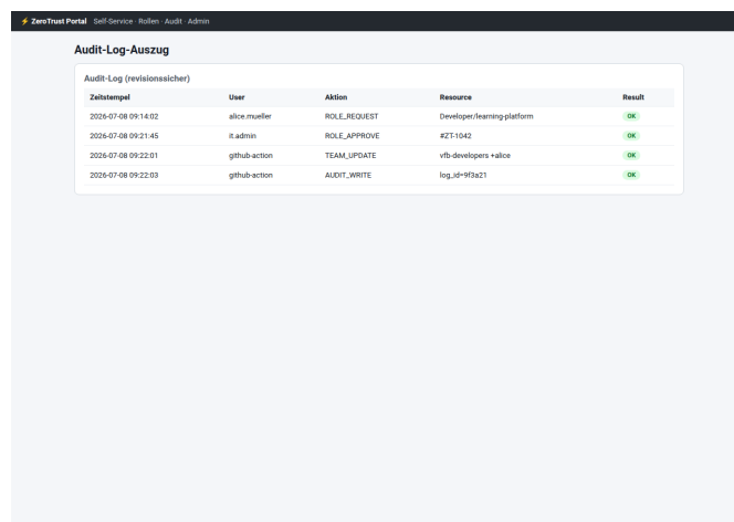
Abbildung 24: Audit-Log-Auszug (Revisionssicherheit)
