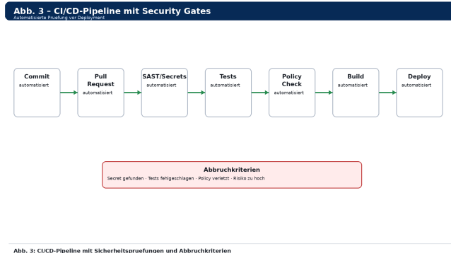
Abbildung 18: CI/CD-Pipeline mit Security Gates
