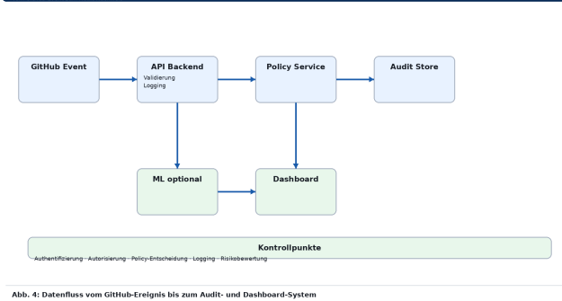
Abb. 4: Datenfluss vom GitHub-Ereignis bis zum Audit- und Dashboard-System
