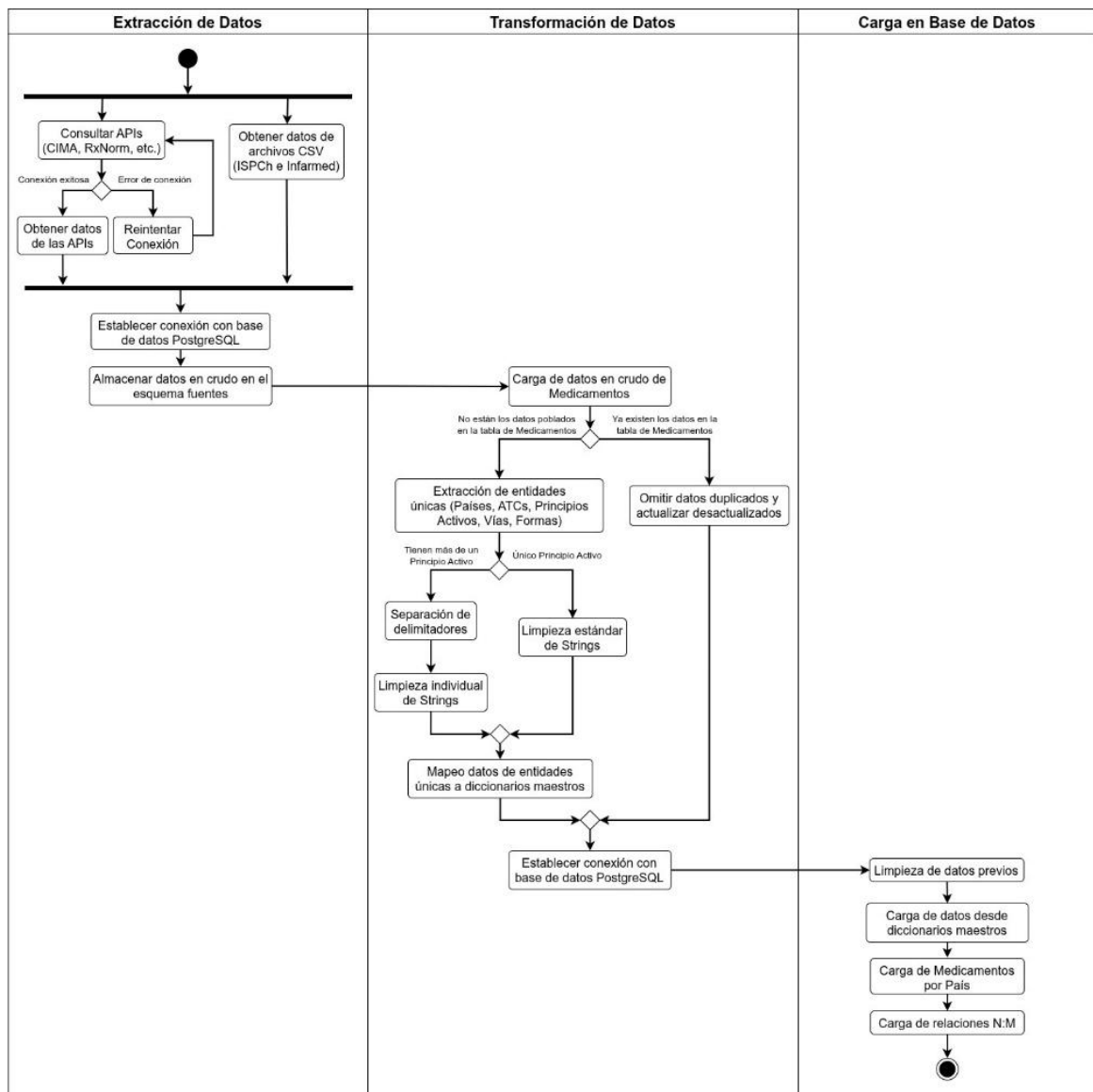
Figura 8.2: Diagrama de Actividad sobre el proceso ETL
