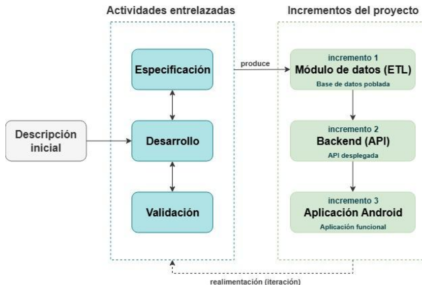
Figura 4.1: Modelo de desarrollo incremental e iterativo aplicado al proyecto (Adaptado de [5])
