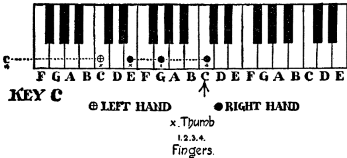
FIG. 1.—First chord.
