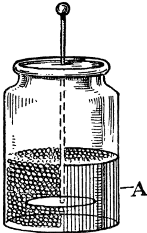
FIG. 3.—Leyden jar.
