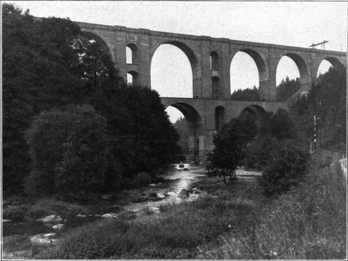
Abb. 1. Elstertalbrücke bei Jocketa
