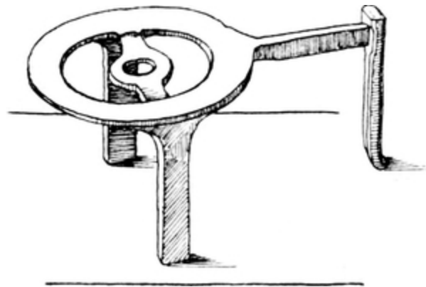
Fig. 20. Erweiterter Dreifuß [H. G. 5735.]
