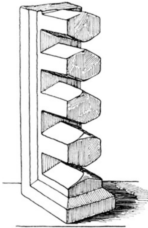
Fig. 26. Steinerne Pfannenhälter in der Küche des Museums.
