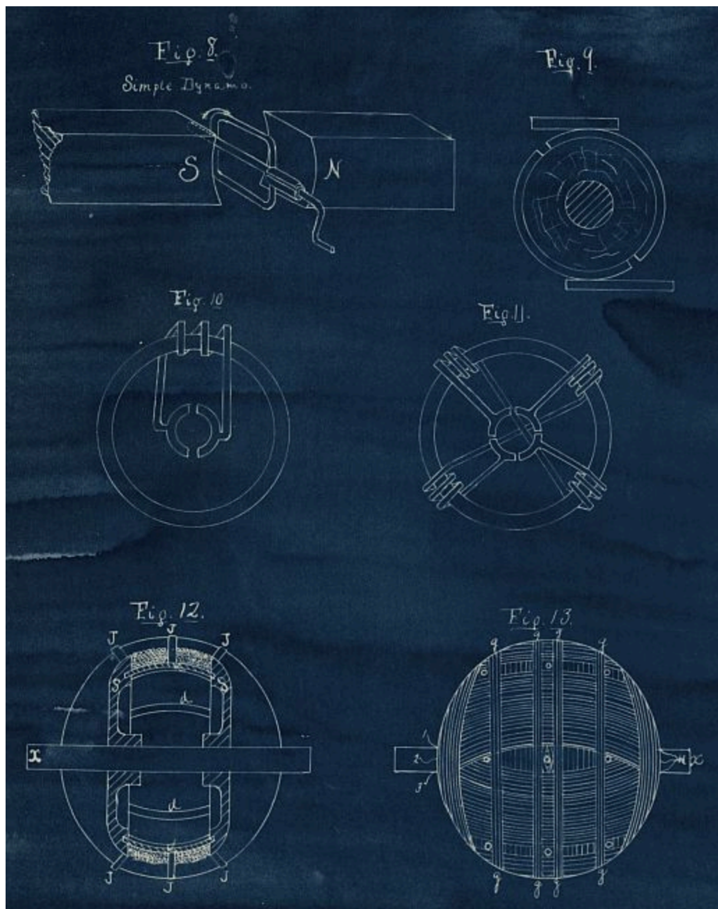
Fig. 8. Simple Dynamo.
