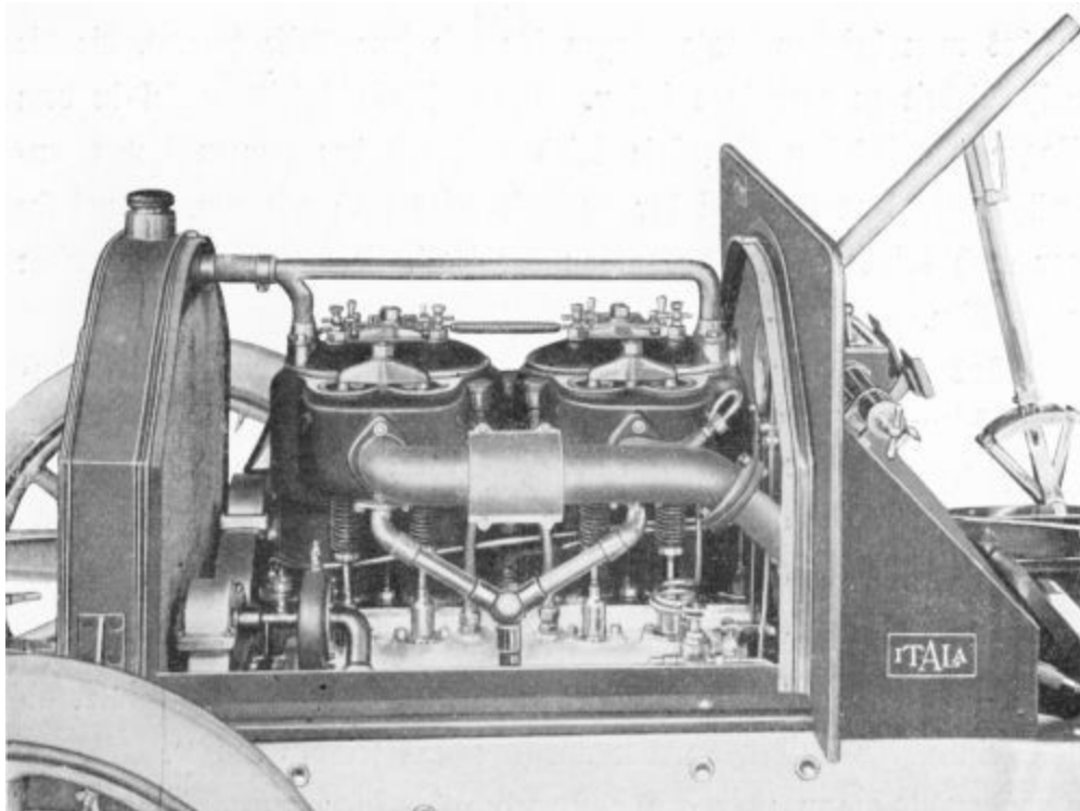
Auspuffseite.
