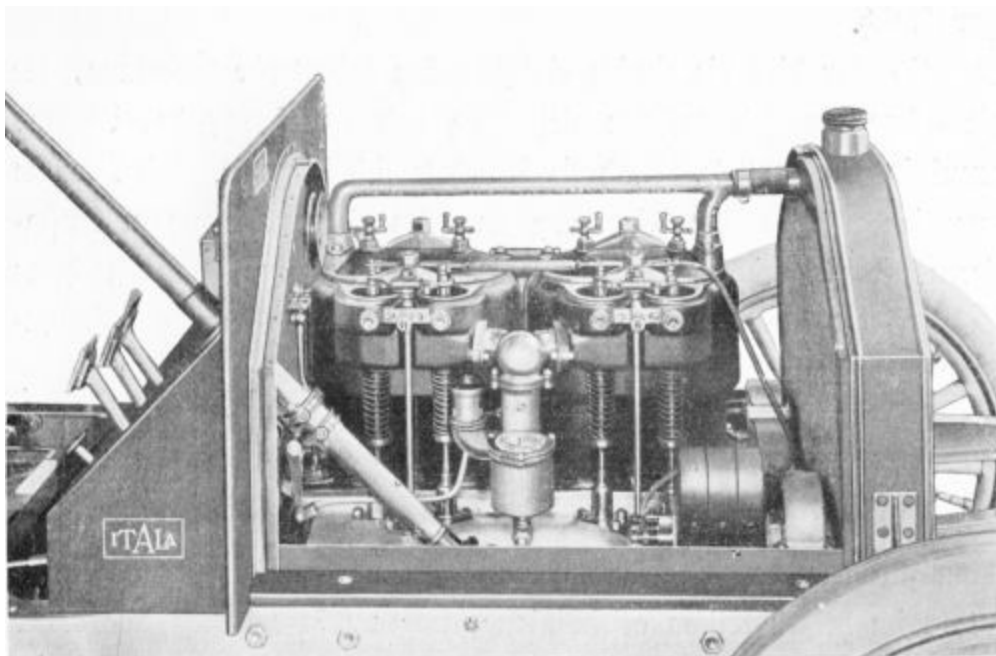
Ansaugseite.
