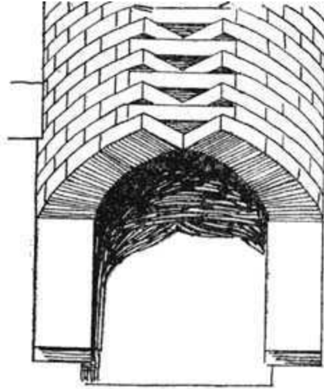
FIG. 19. (Place, Nineveh , Pl. 38.) FIG. 20. (Place, Nineveh , Pl. 38.)
