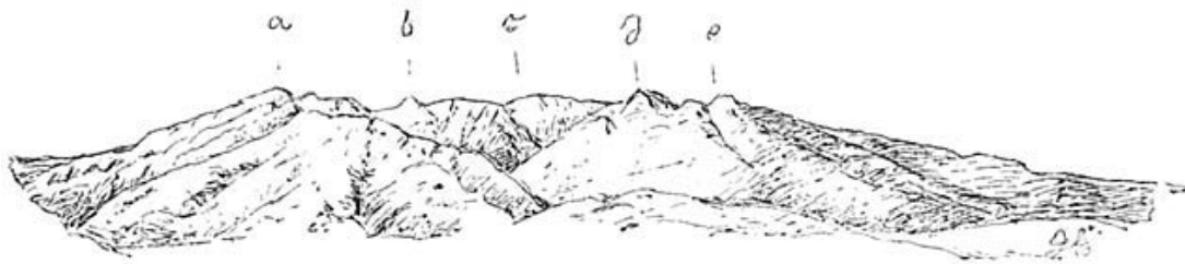
Die Spitze a liegt von Tibi gesehn S. 49°7; b 54°8; d 64°2; e 67° W.; die Einsenkung c S. 59°5 W.
