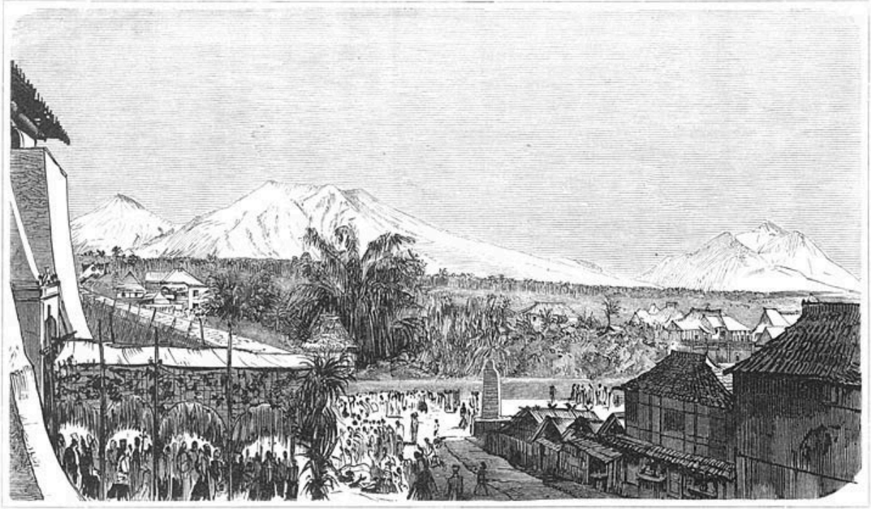
Vulkan Majaijai und San Cristobal.
