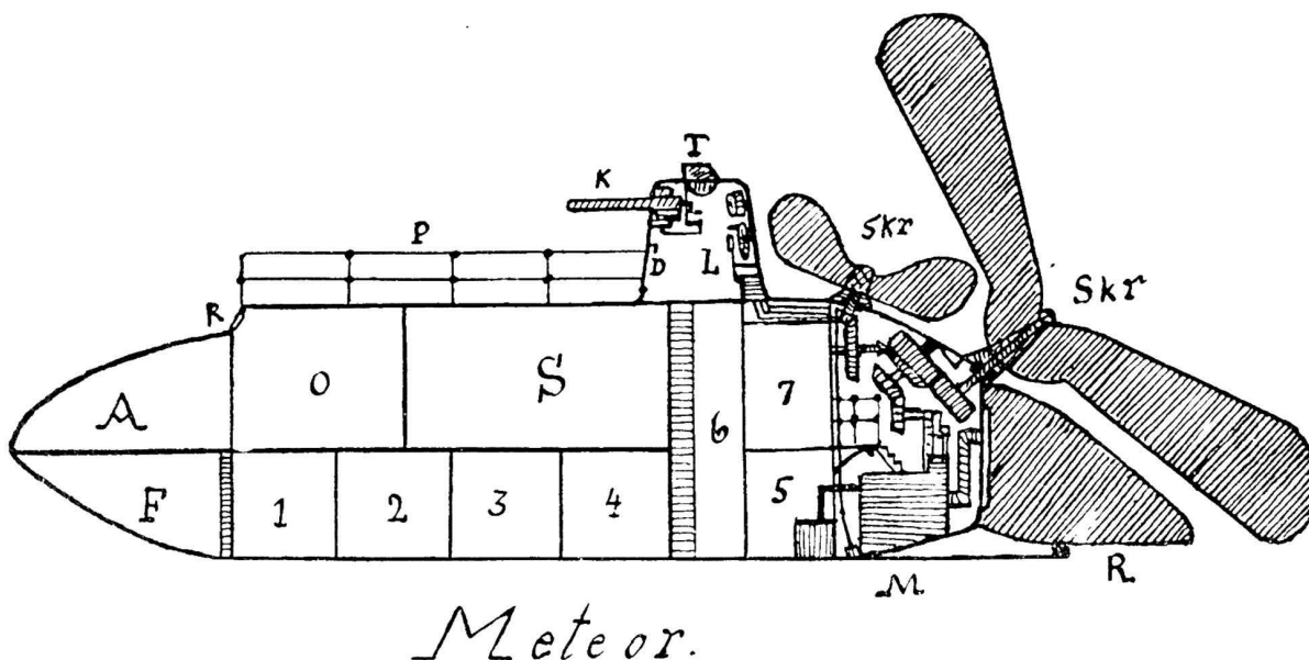
Hydes Tegning af Luftskeibet, set i Gennemsnit.
