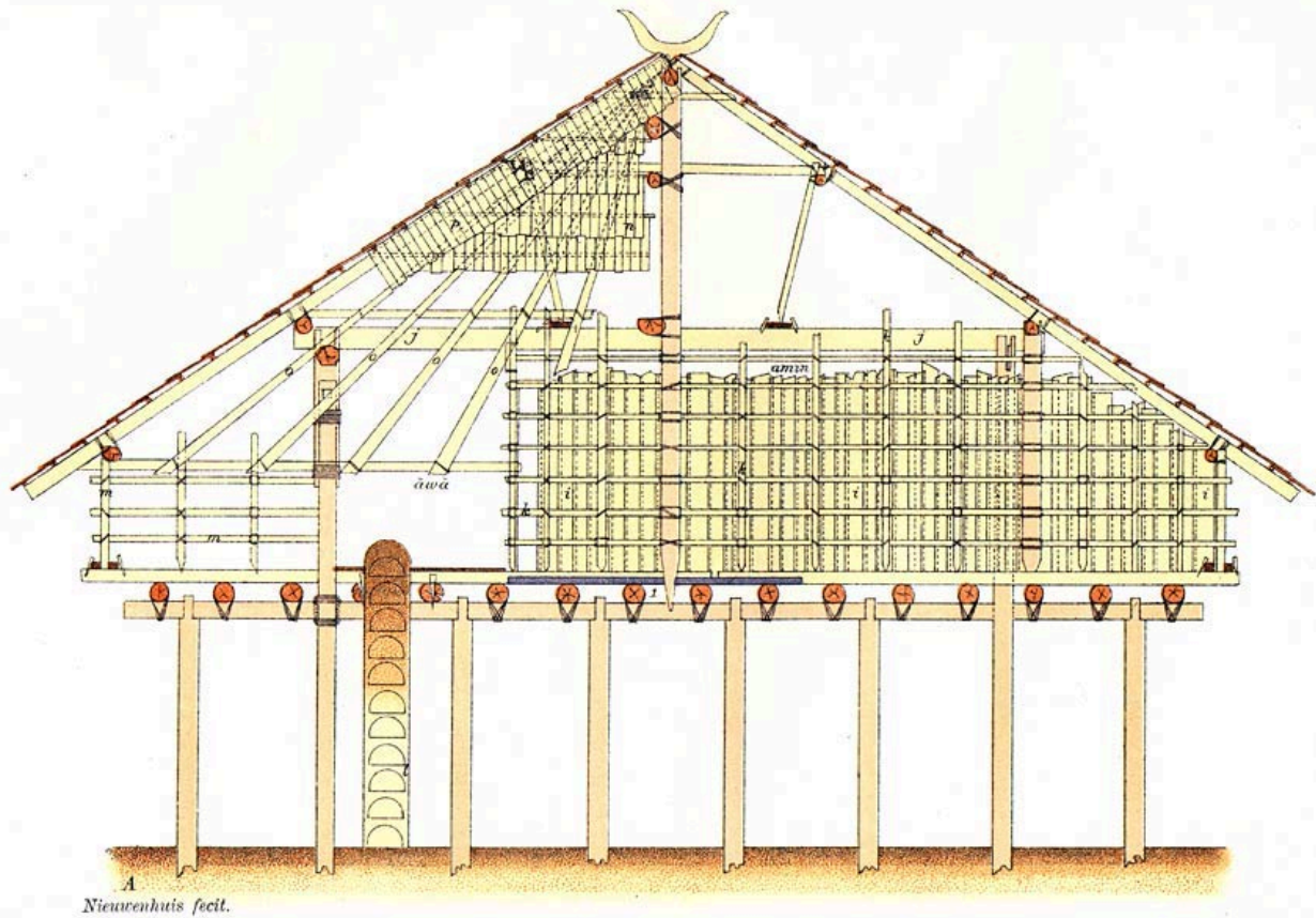
Seitenansicht eines panjin -Hauses.
