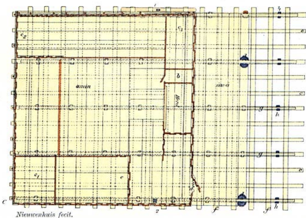
Grundriss des panjin -Hauses.
