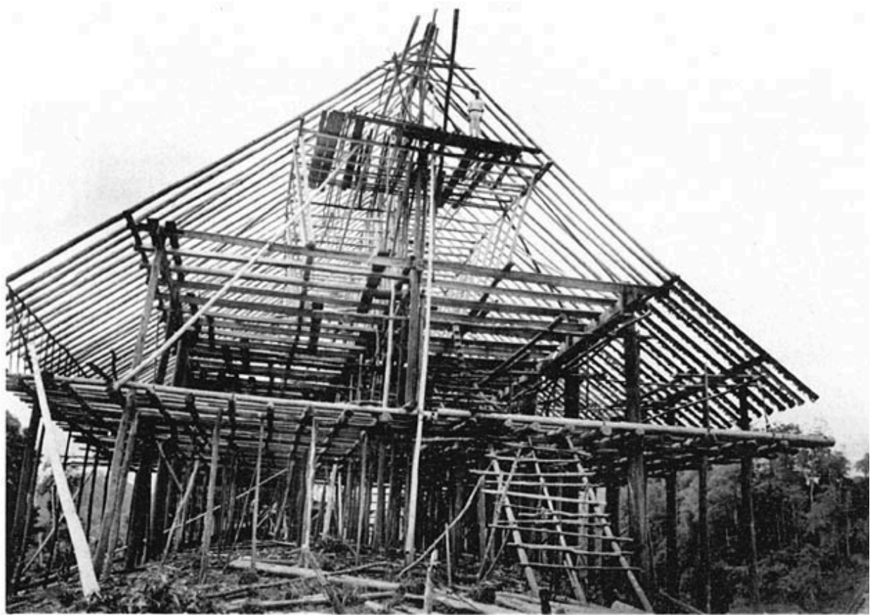
Gerüst von KWING IRANGS Haus.
