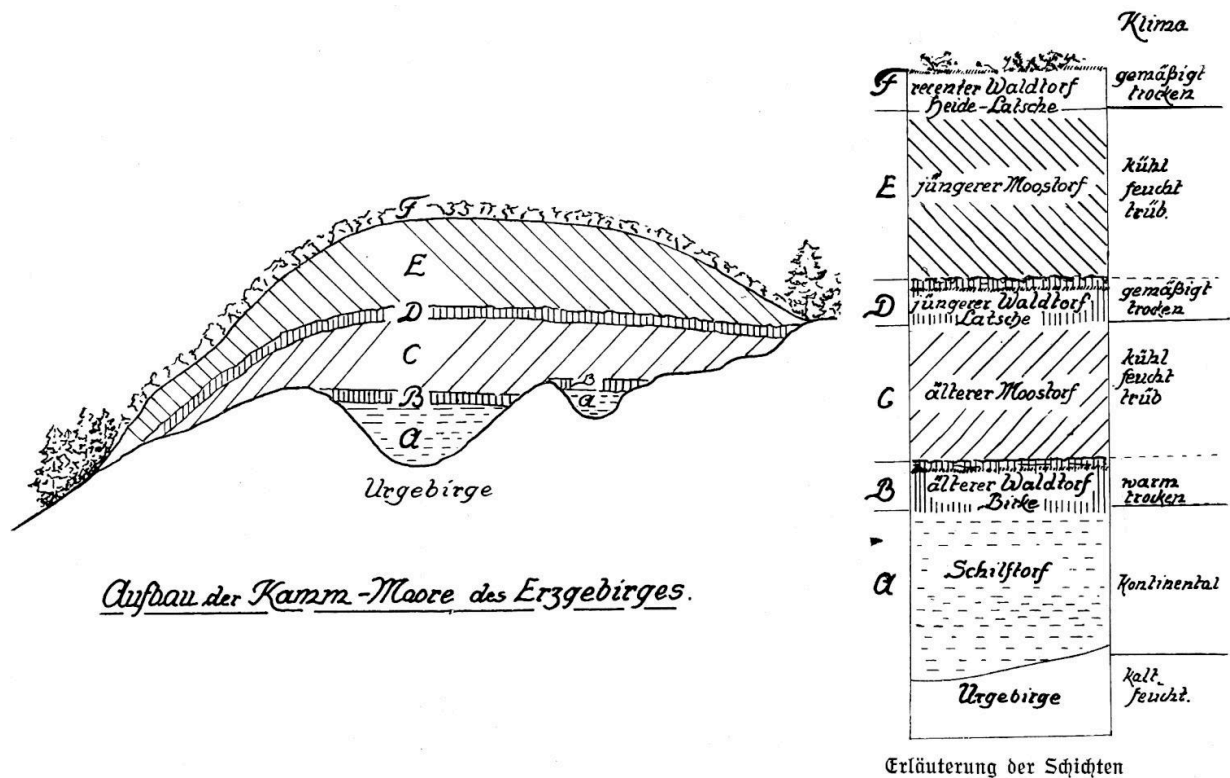
Abb. 14. Aufbau der Kamm-Moore des Erzgebirges. (Moorprofil nach Prof. Schreiber, Sebastiansberg)
