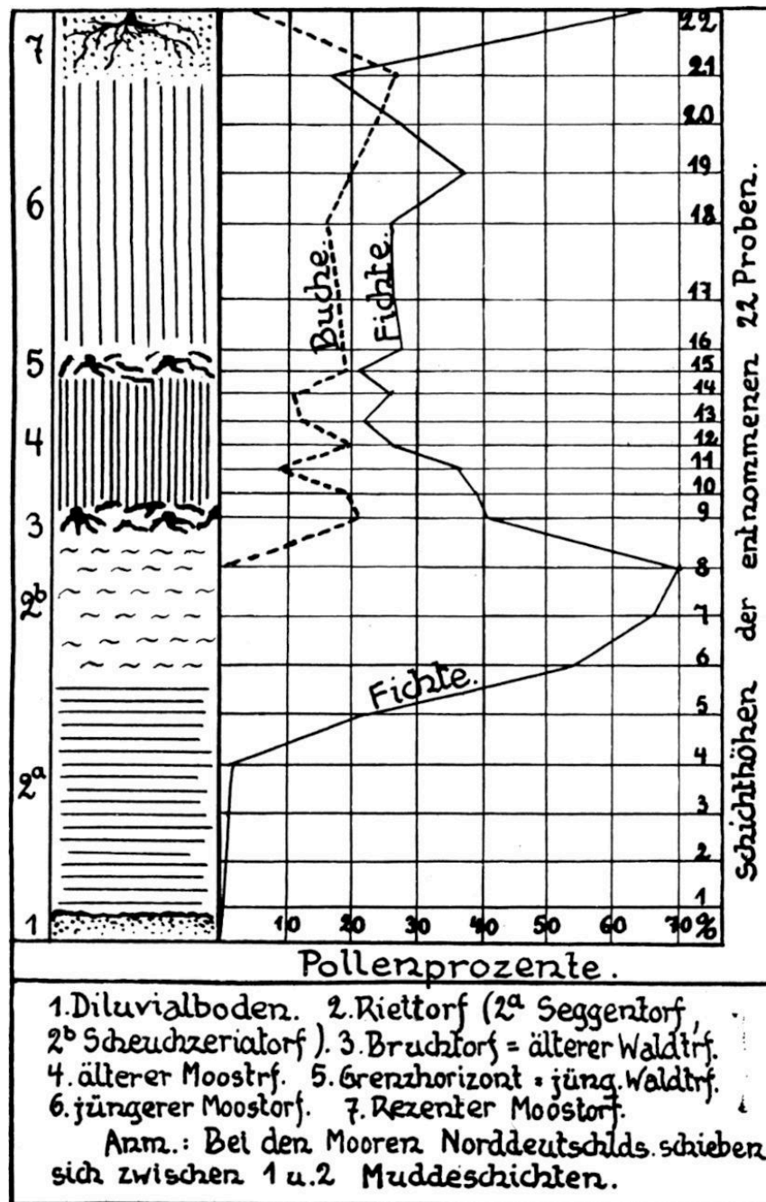
Abb. 20 Übersichtliche Darstellung der Ergebnisse von Pollenanalysen nach Rudolph und Firbas
