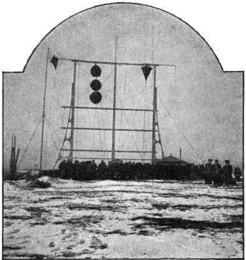
Het seintoestel bij het Noorderhoofd. ( vergroting 841×894, 167kb )
