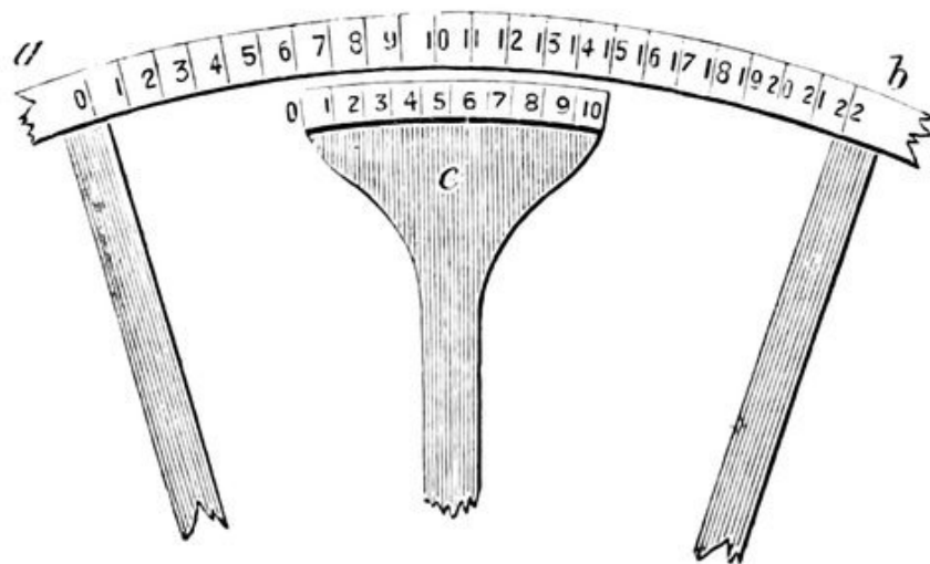
FIG. 102.—The Vernier.
