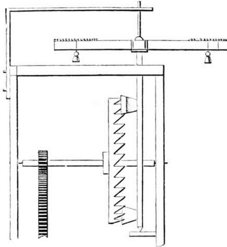
FIG. 85.—Ancient Clock Escapement.
