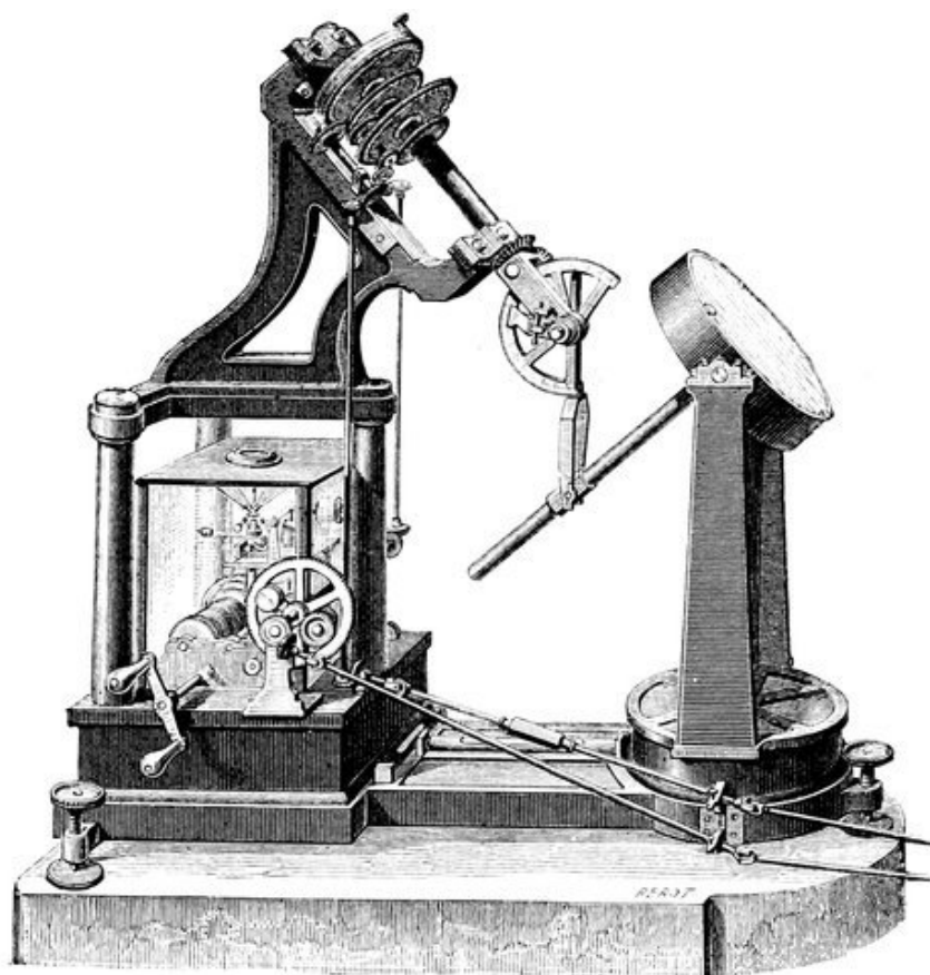
FIG. 156.—Foucault's Siderostat.
