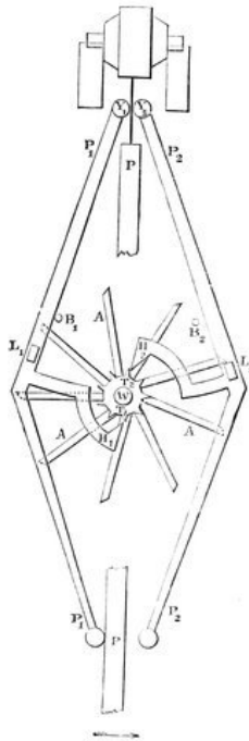
FIG. 95.— Gravity Escapement (Bloxam).
