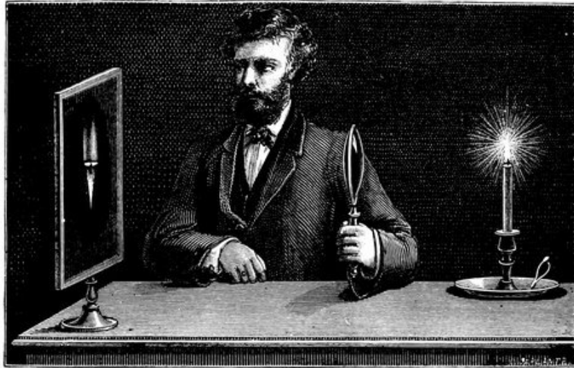
FIG. 29.—Conjugate Images.
