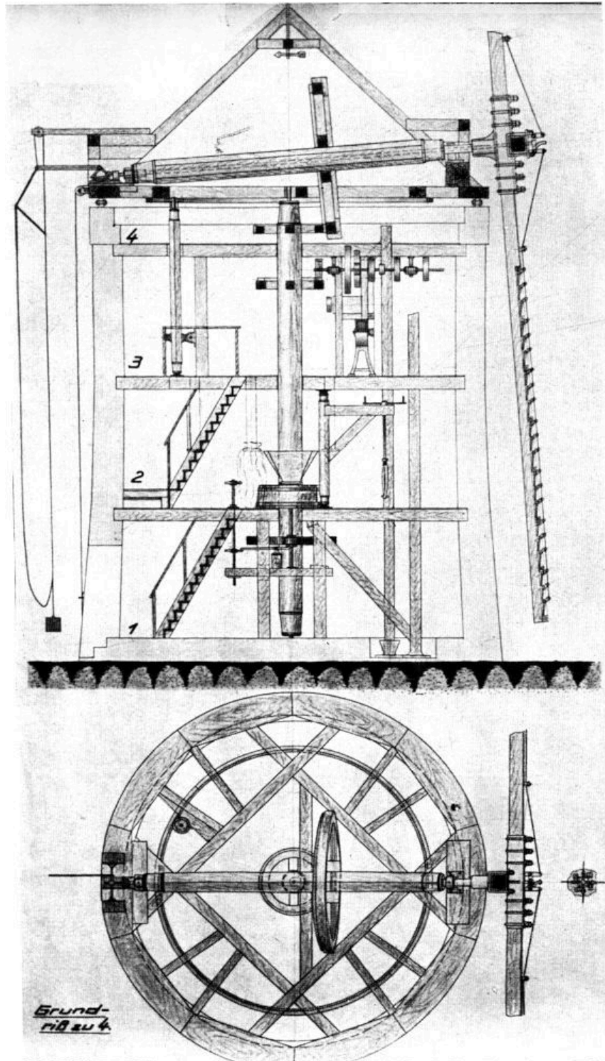
Das Innere der Syrauer Windmühle
