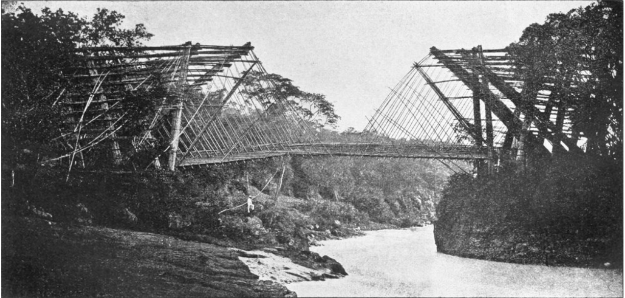
Fig. 16. Eine Hängebrücke aus Bambus bei Bandjar im Serajo-Thal (Bezirk Bandjarnegara).
