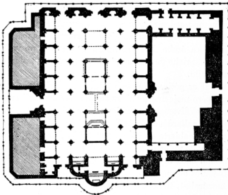
Planta de la Catedral de Sevilla.
