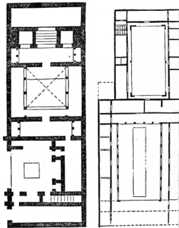
Planta de los Baños.
