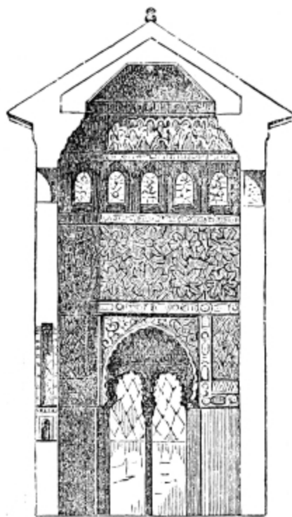
Sección de la Torre de Said.
