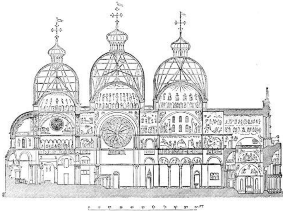
416. Section of St. Mark's, Venice. (From 'Chiesi Principali di Europa.')
