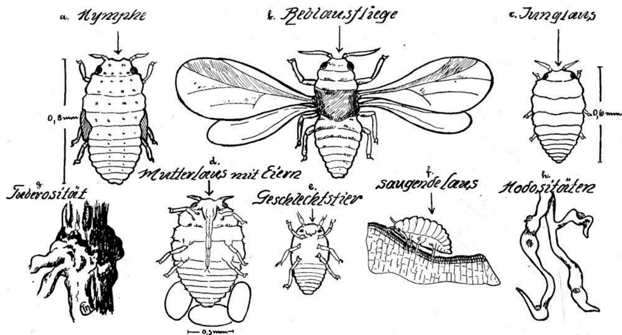
Abb. 2 Die Vernichterin des Lößnitzer Weinbaues: die Reblaus ( Phylloxera vastatrix ) in ihrer Entwicklung
