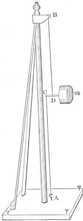
Fig. 82.—Horizontal Pendulum.
