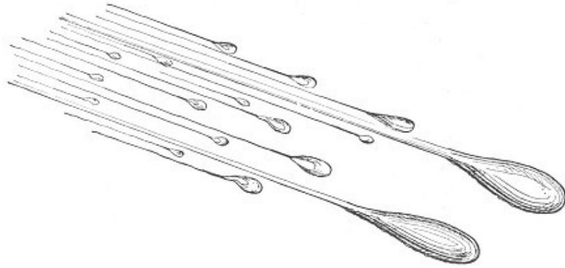
Fig. 49.—Bolides.
