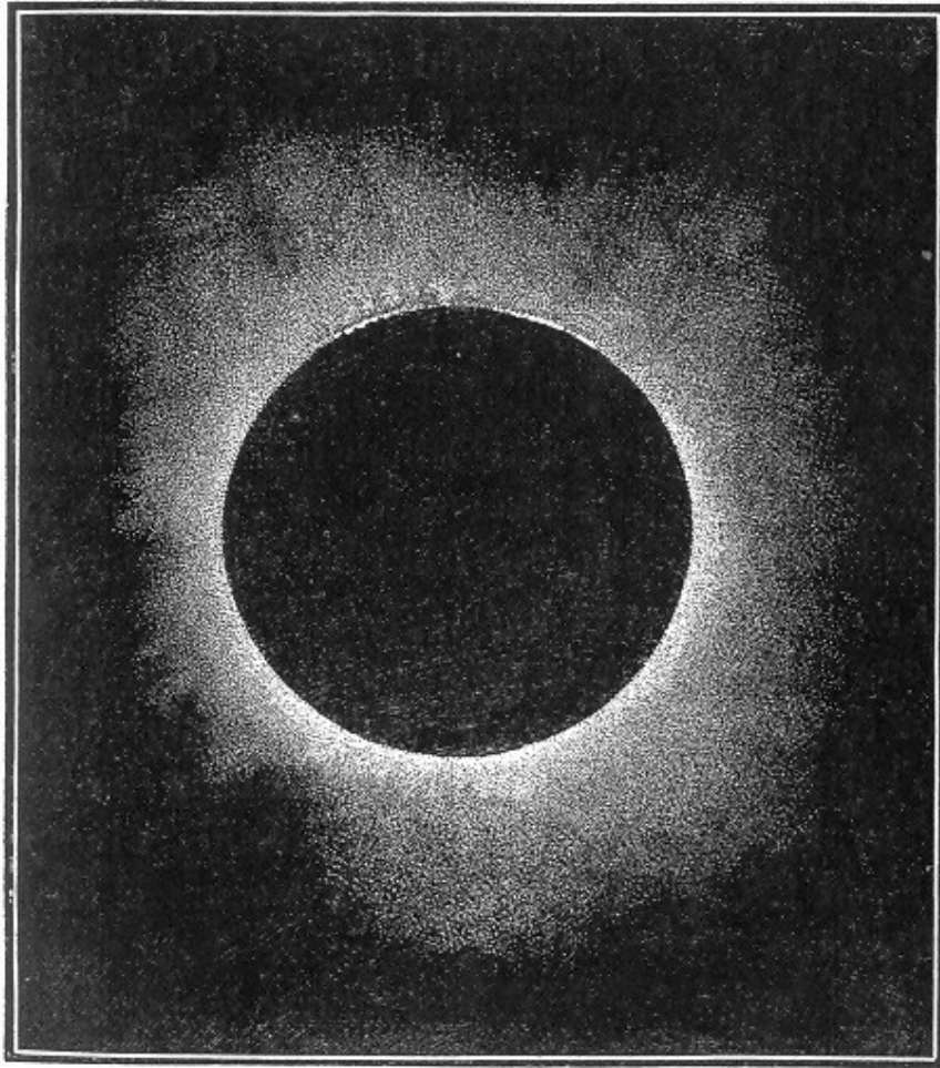
Fig. 33.—The Corolla in 1878, Colorado.
