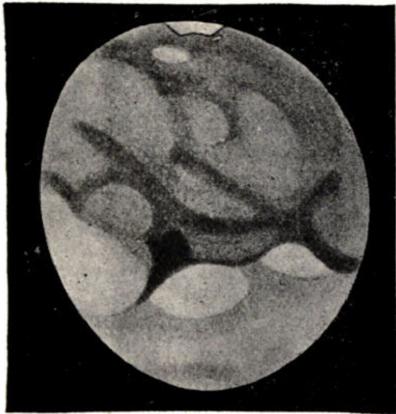
Fig. 52.—Drawing of Mars (August 16th, 1894).
