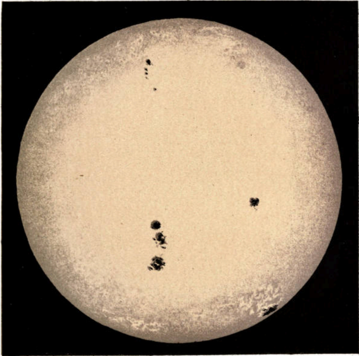
PLATE A. THE SUN.
