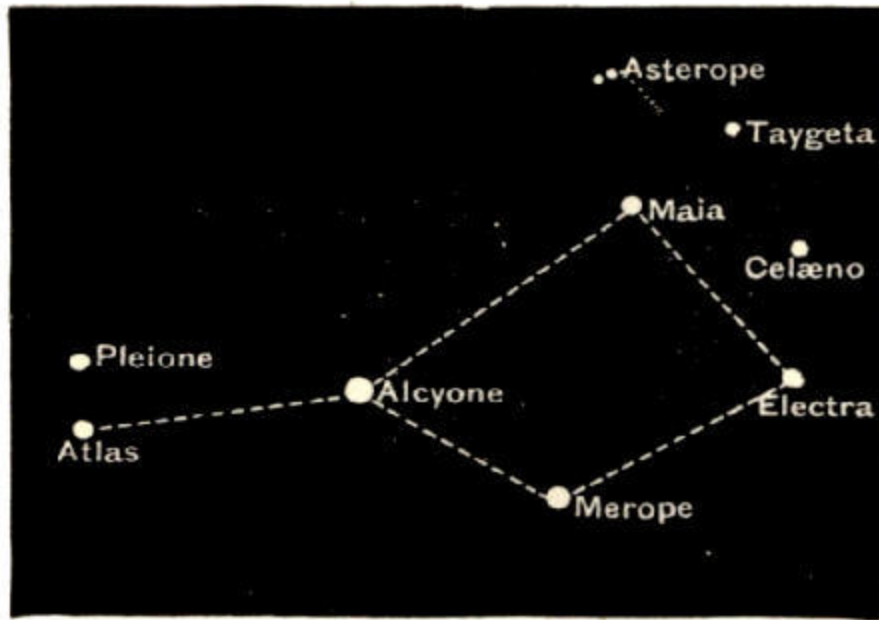
Fig. 84.—The Pleiades.
