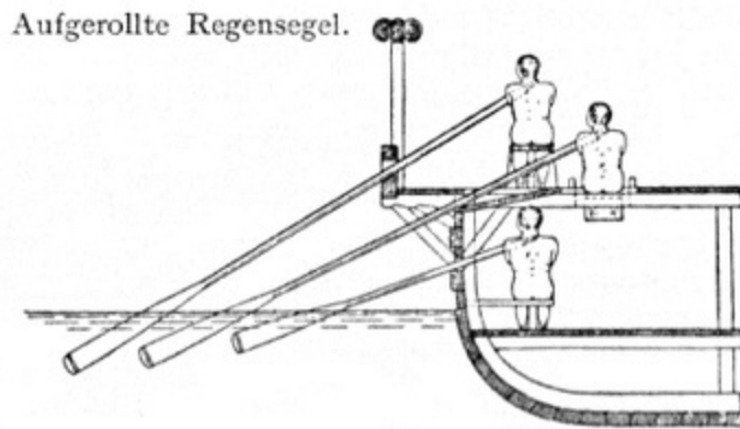
Triere. Teil des Querschnittes. Zeichnung der Rudereinrichtung nach R. Haack.
