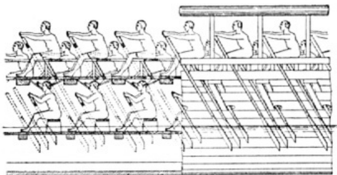
Triere, Teil des Längsschnittes.
