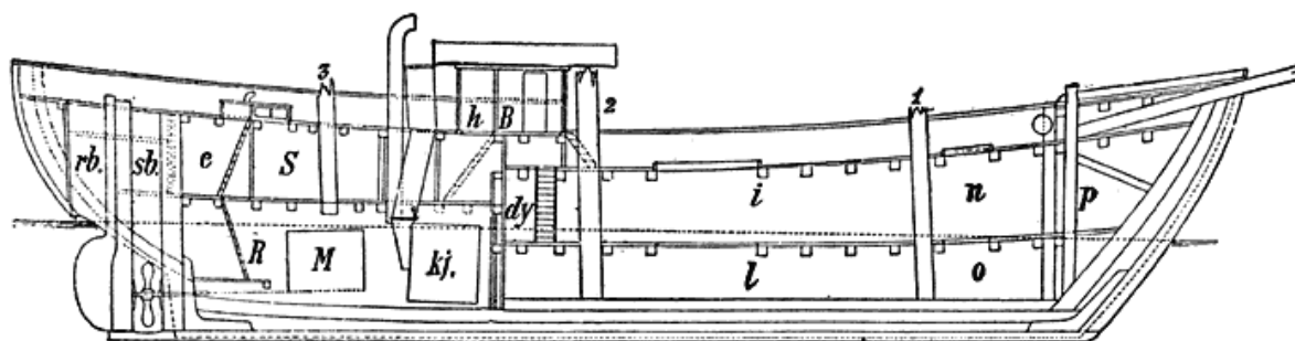
Fig. 1. Longitudinal section.
