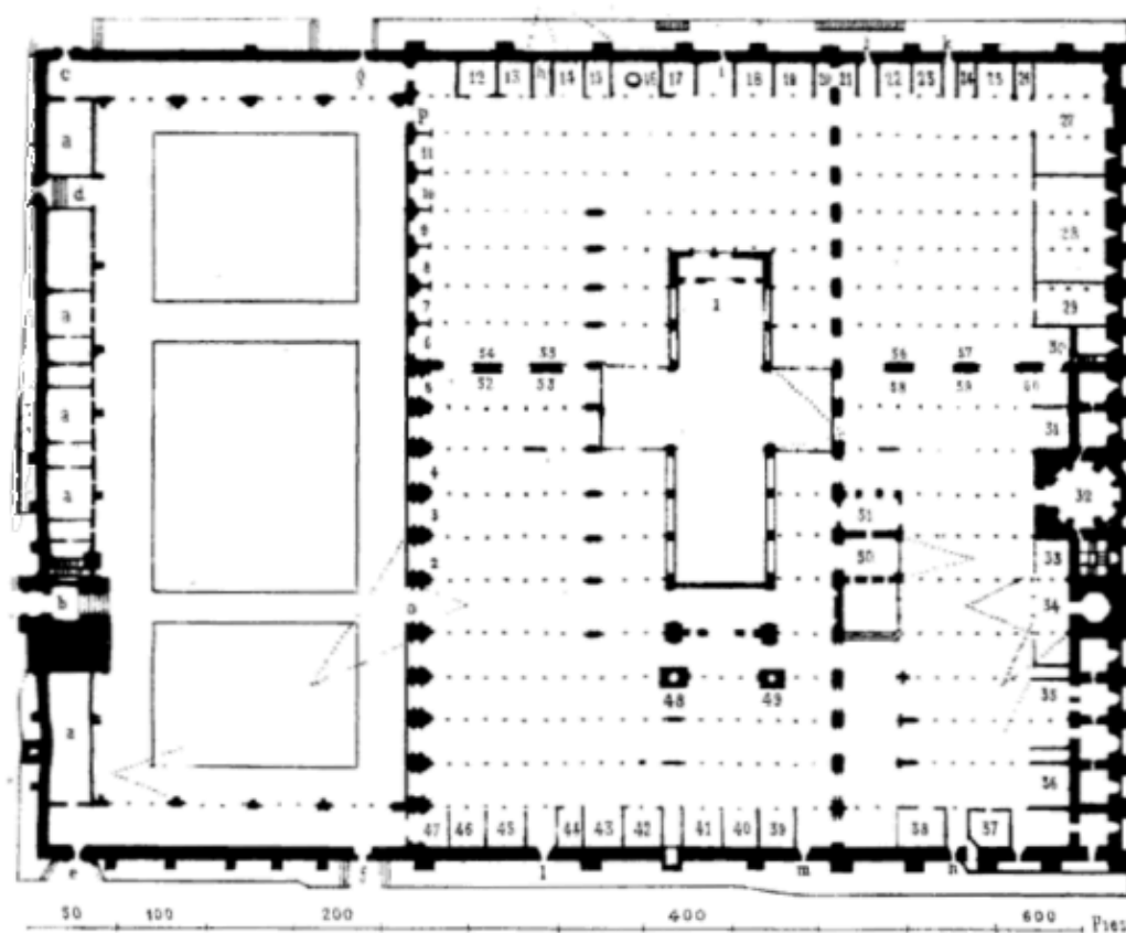
PLANTA DE LA CATEDRAL DE CÓRDOBA.
