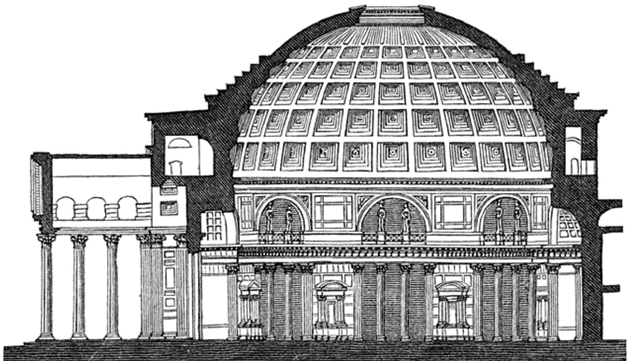
Pantheon, in doorsnede van binnen gezien.
