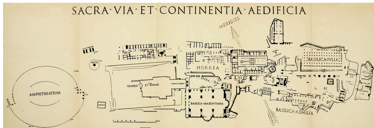
Tavola 96. — Rilievo grafico generale dello stato attuale del Foro Romano, risultante dalla connessione a penna nella scala di 1:500 dei rilievi altimetrici parziali, eseguiti l'anno 1900 dagli alunni della R. Scuola d'applicazione degli ingegneri in Roma nell'area compresa tra il Colosseo e il Tabularium . (Cfr. Notizie degli Scavi , giugno 1900, pag. 220 e segg.).
