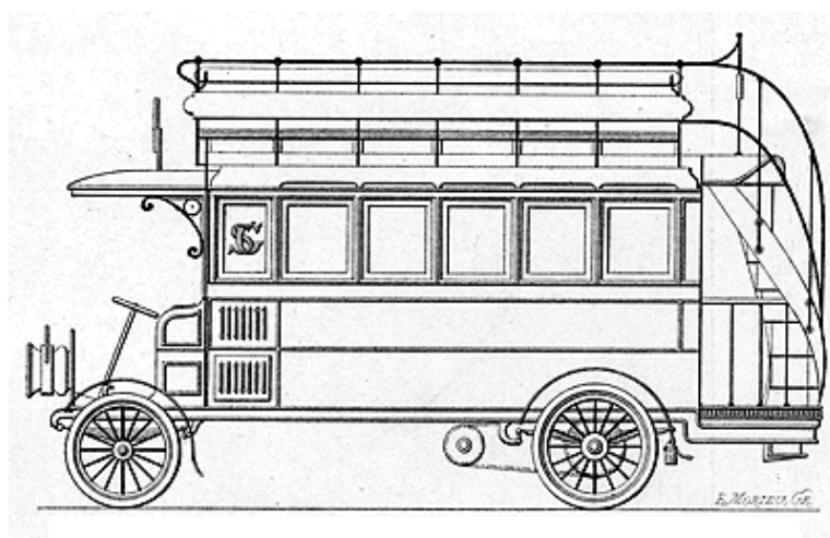
L'omnibus automobile de demain, actuellement en construction.
