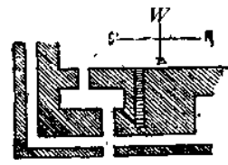
Fig. 31. --Plan of gate, fortress of Kom el Ahmar.
