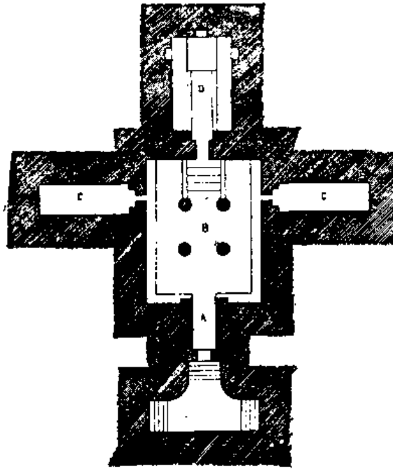
Fig 88 .--Plan of Speos, Kalaat Addah, Nubia.
