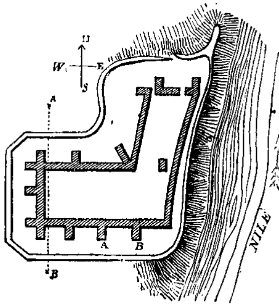
Fig. 35.--Plan of fortress of Semneh.
