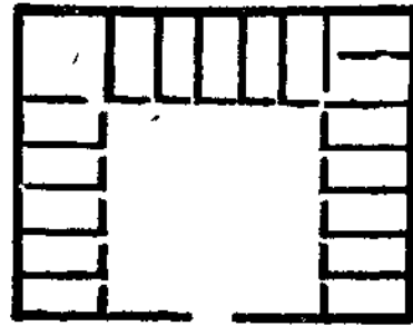
Fig. 5. --Plan of house, Medinet Habû.
