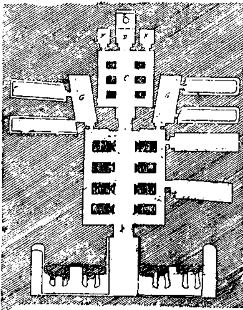
Fig 90 .--Plan of the Great Speos, Abû Simbel.
