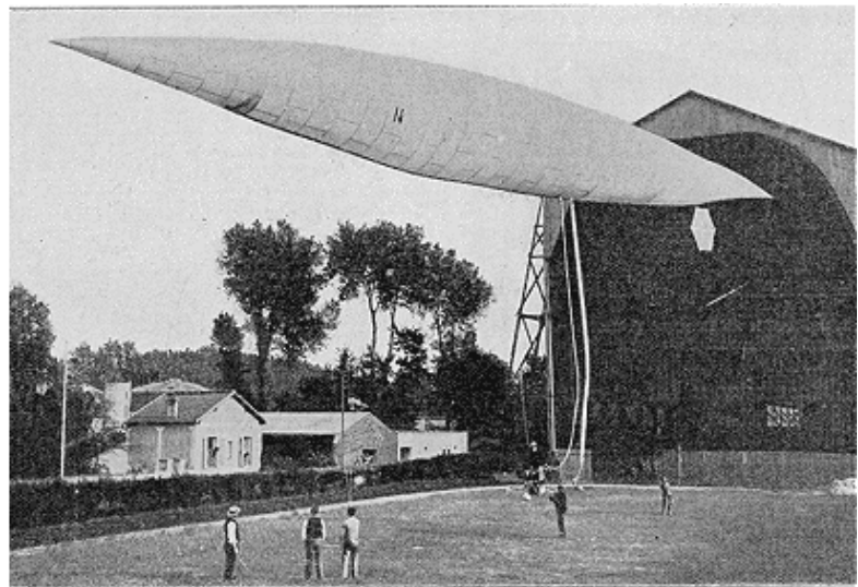
M. Santos-Dumont dans la nacelle de son nouveau dirigeable.
