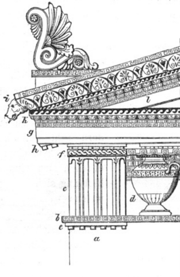
Fig. 36. Dorischer Oberbau.
