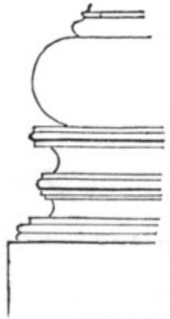
Fig. 37. Spira ionica.
