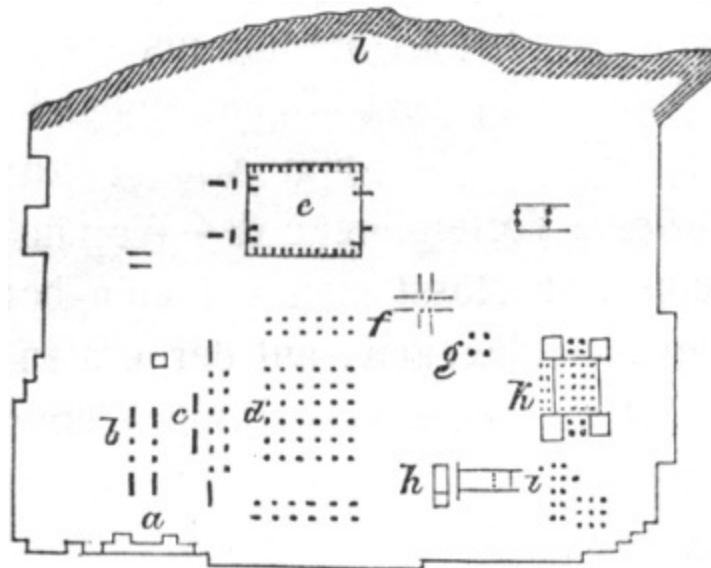
Fig. 23. Grundriss von Tschil-Minar.
