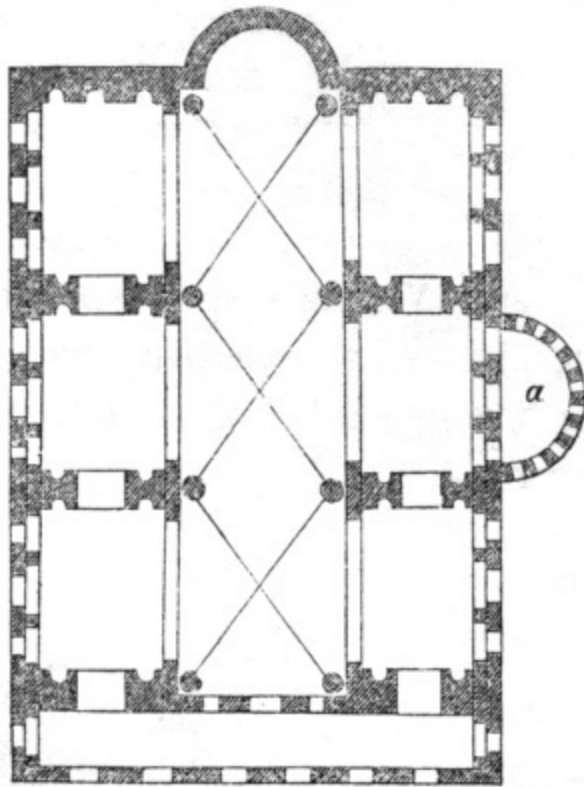
Fig. 51. Basilika des Maxentius.
