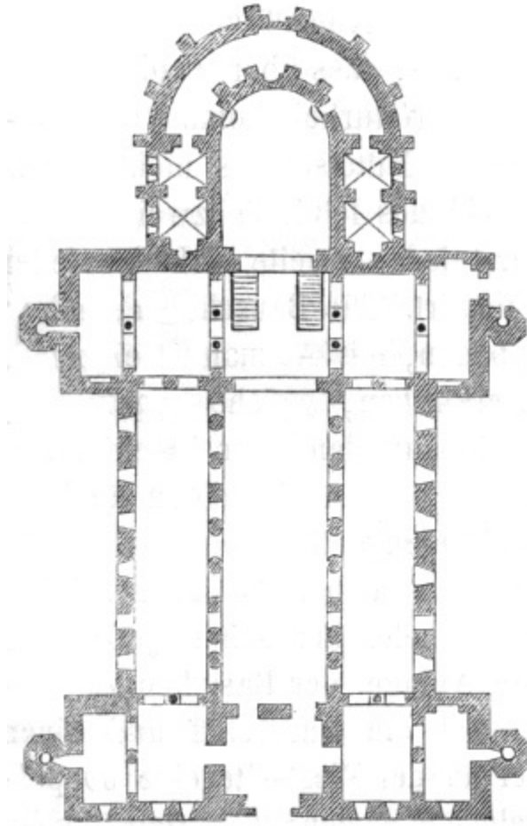
Fig. 85. Michaeliskirche in Hildesheim.
