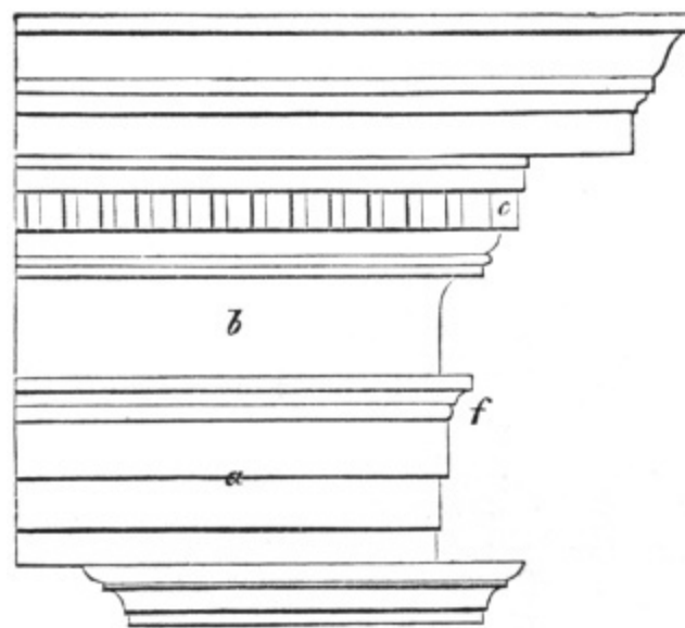
Fig. 39. Ionischer Oberbau.
