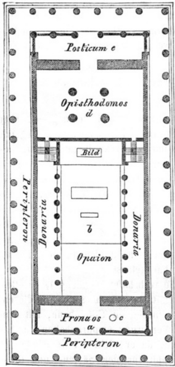
Fig. 32. Grundriss des Parthenon.
