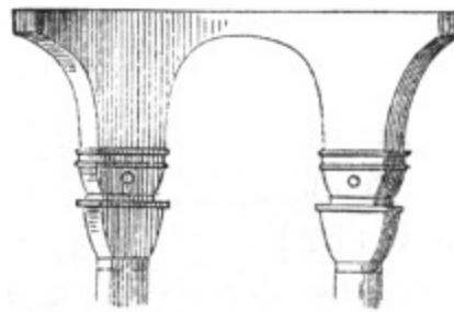
Fig. 57. Ravennatischer Bogen.
