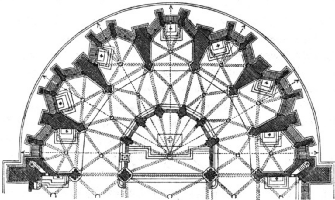
Fig. 78. Chorhaupt vom Kölner Dome.
