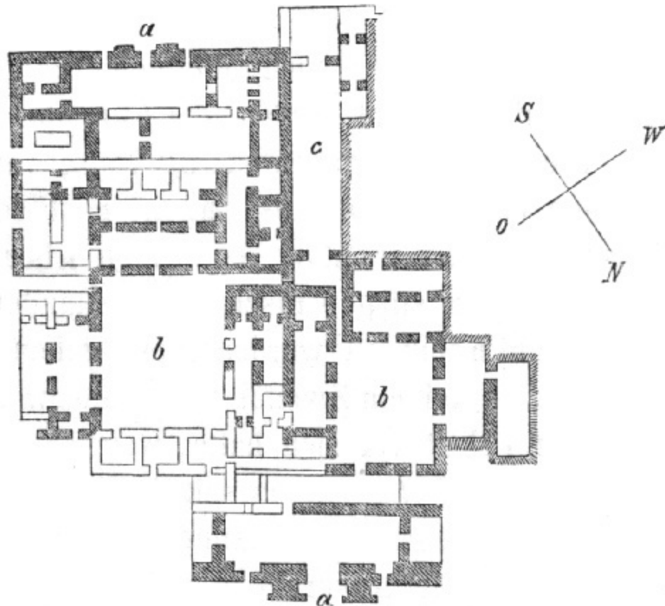
Fig. 15. Plan des Palastes von Kuyundschik.
