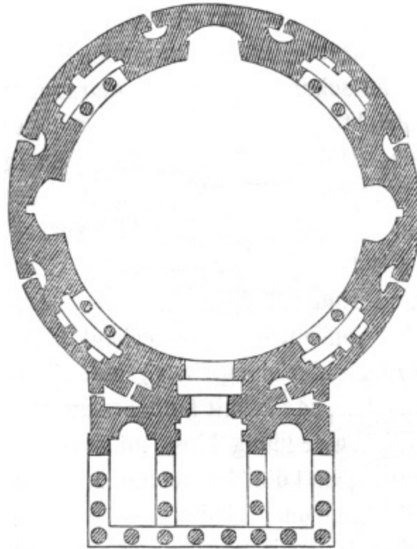
Fig. 48. Grundriss des Pantheon.
