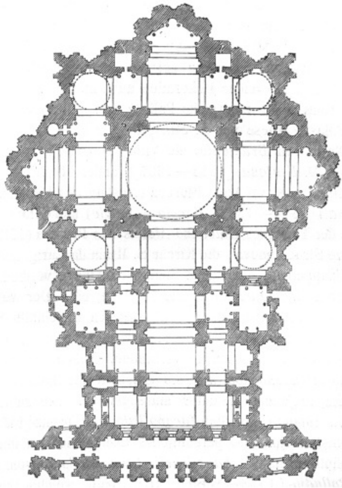
Fig. 89. Grundriss der Peterskirche.
