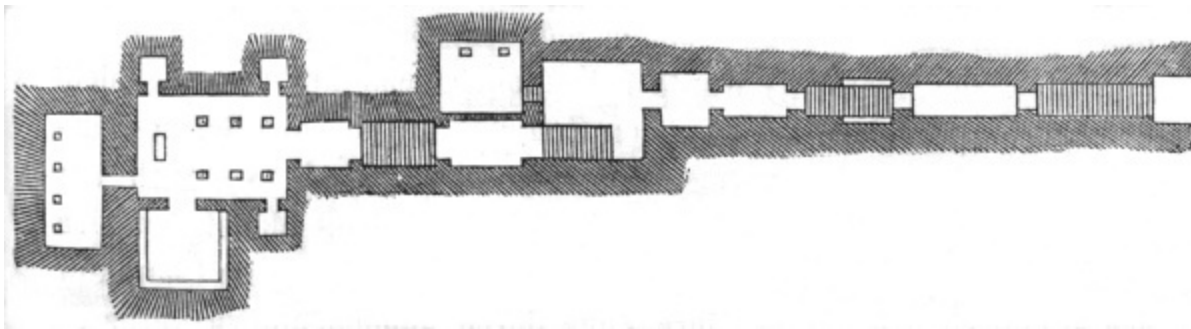
Fig. 28. Felsgrab des Merenptah in Theben.
