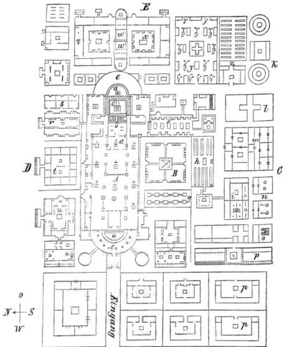
Fig. 66. Grundriss des Klosters S. Gallen.
