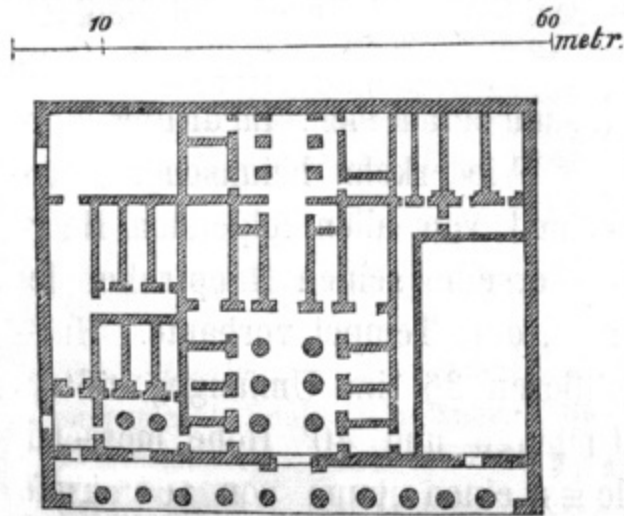
Fig. 27. Tempel von Qurna.
