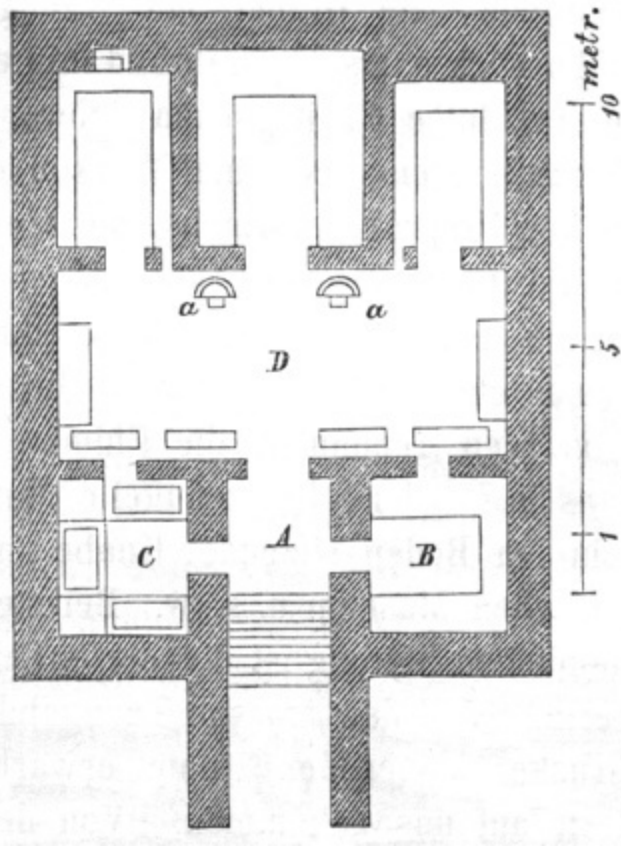
Fig. 46. Grab aus Caere.
