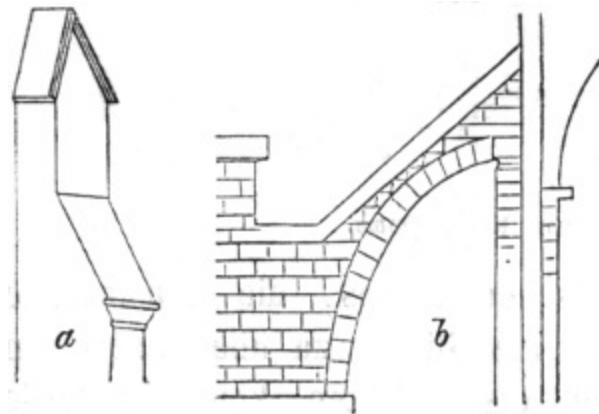
Fig. 81. Strebepfeiler und Strebebogen.
