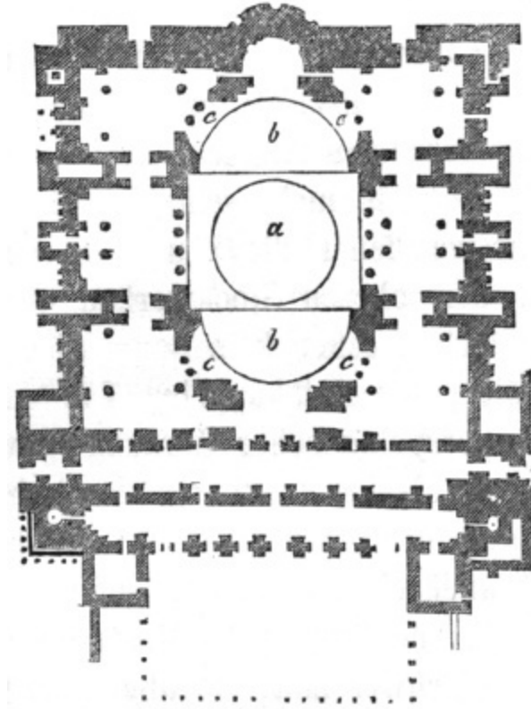
Fig. 58. Grundriss der Sophienkirche.
