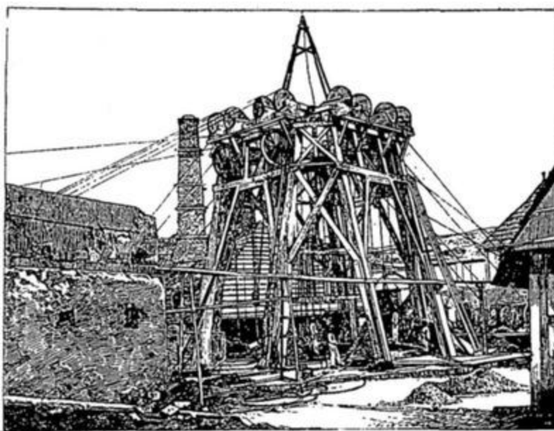
MEXIQUE.—GUANAJUATO.—PUITS D'EXTRACTION DE LA MINE VALENCIANA. (600 MÈTRES DE PROFONDEUR.)
